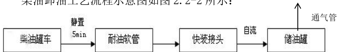
图 2.2-2 柴油卸油工艺流程示意简图
