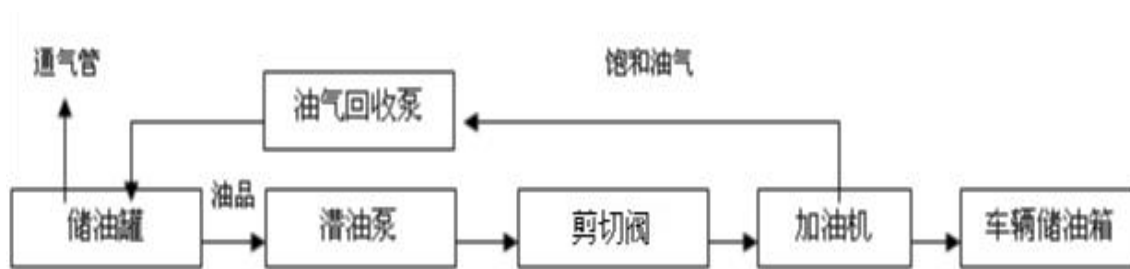
图 2.2-3 汽油加油工艺流程示意简图
