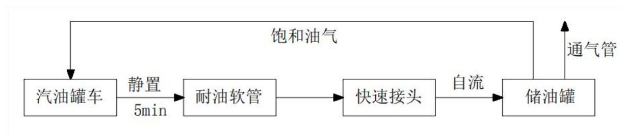
图 2.2-1 汽油卸油工艺流程示意简图
