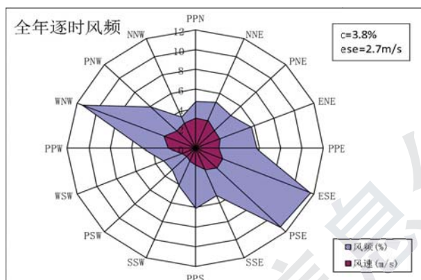
(a) 全年风玫瑰图
