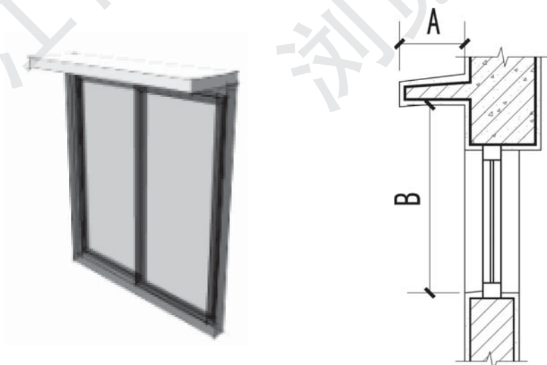
图 A. 3. 1-1 水平式外遮阳的特征值
