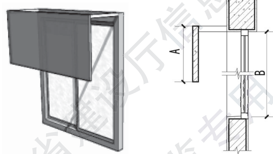
图 A. 3. 1-3 挡板式外遮阳的特征值
