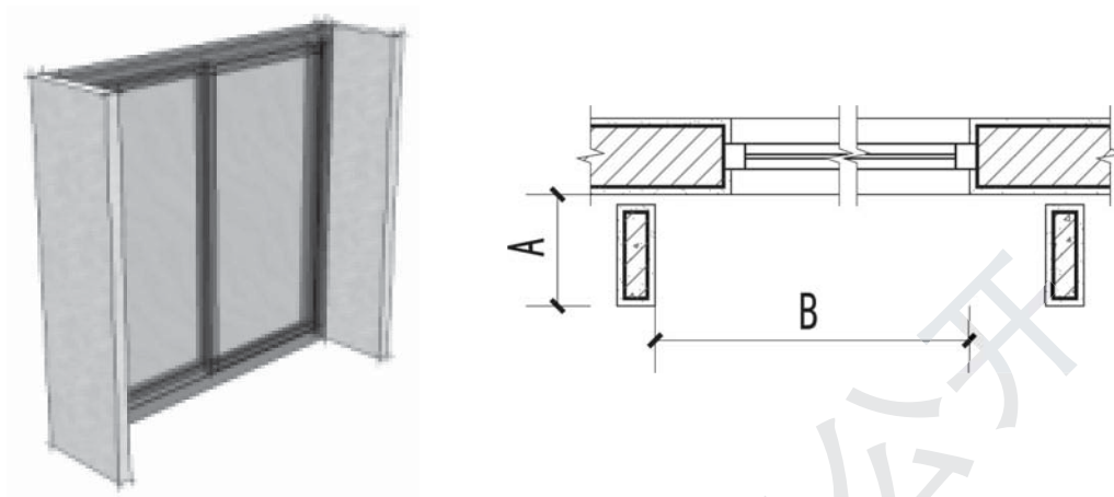
图 A. 3. 1-2 垂直式外遮阳的特征值
