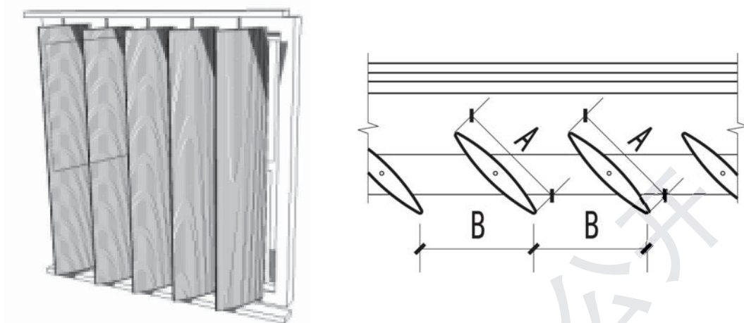
图 A. 3. 1-5 活动竖百叶挡板式外遮阳的特征值
