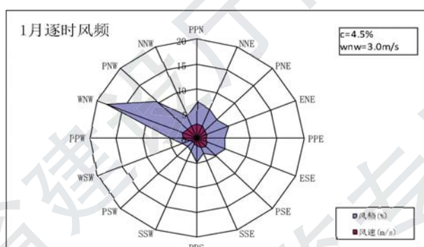
(b) 一月风玫瑰图
