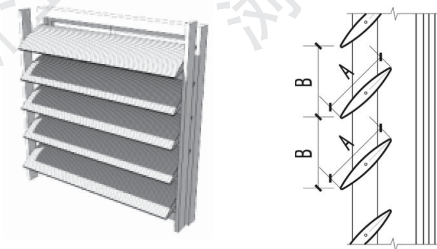
图 A. 3. 1-4 横百叶挡板式外遮阳的特征值
