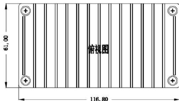
标准型+散热器 116.8*61*32.5mm
