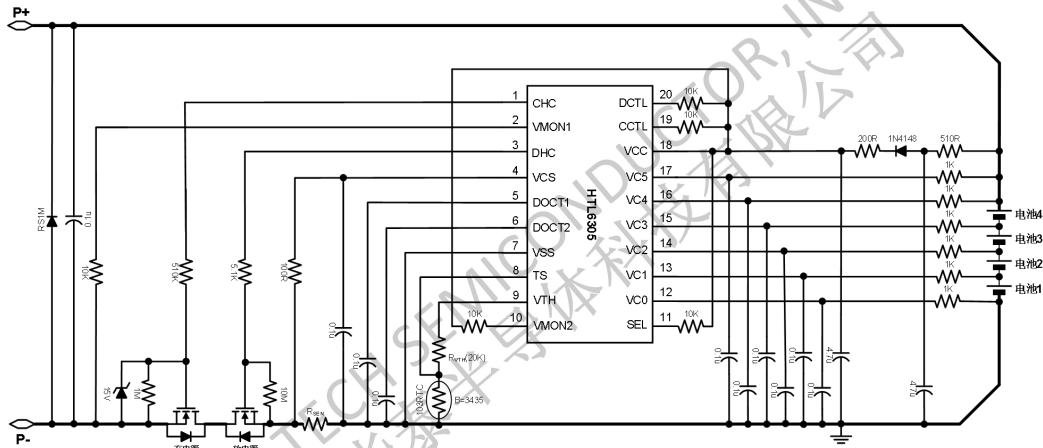
图 4 4 节电池包的 N 型充电管和 N 型放电管的同口典型应用电路图
