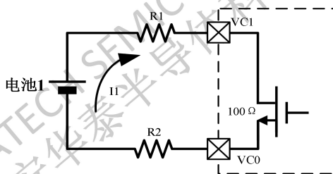
图 9 内部均衡驱动原理图
