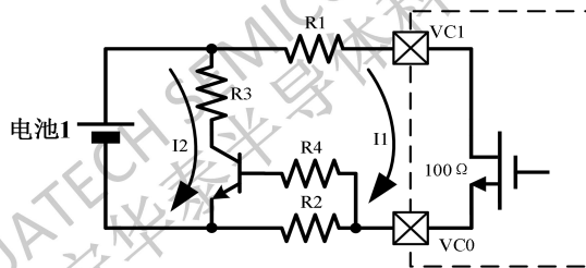
图 10 外部扩展均衡原理图
