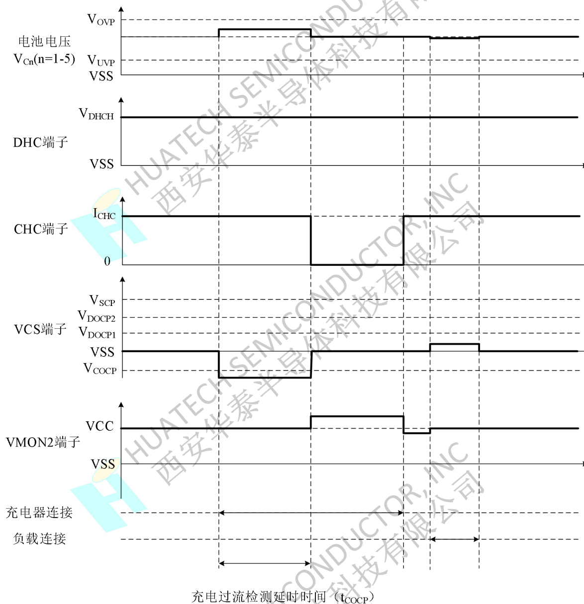
图 16 充电过流检测
