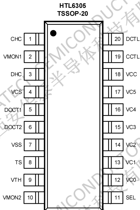
图 7 引脚分布
