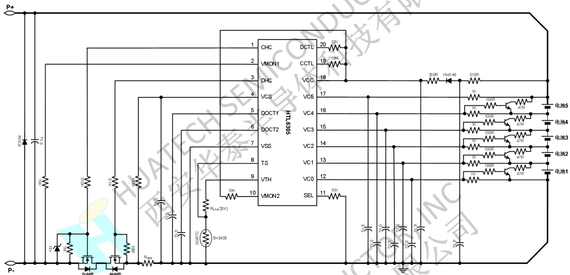
图 5 5 节电池包外部扩展均衡的 N 型充电管和 N 型放电管的同口典型应用电路图
