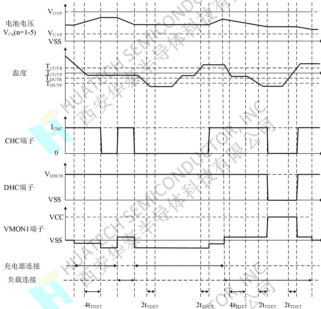
图 18 充放电低温检测
