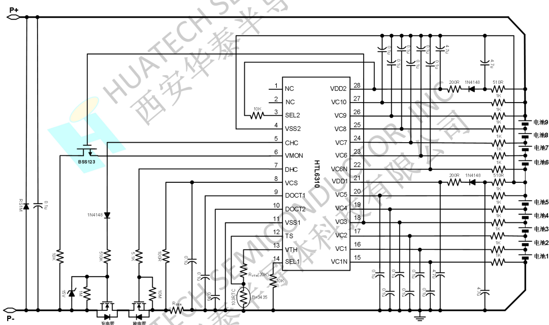
图 3 9 节电池包的 N 型充电管和 N 型放电管的同口典型应用电路图
