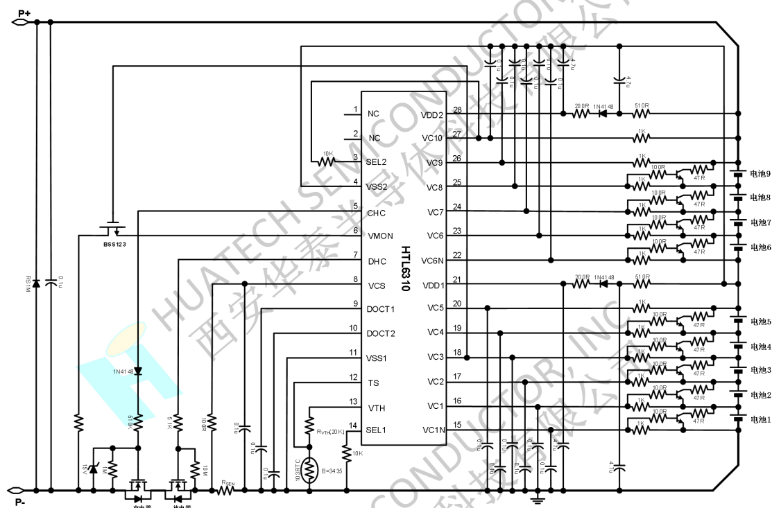
图 6 9 节电池包外部扩展均衡的 N 型充电管和 N 型放电管的同口典型应用电路图
