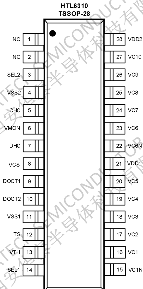
图 7 引脚分布
