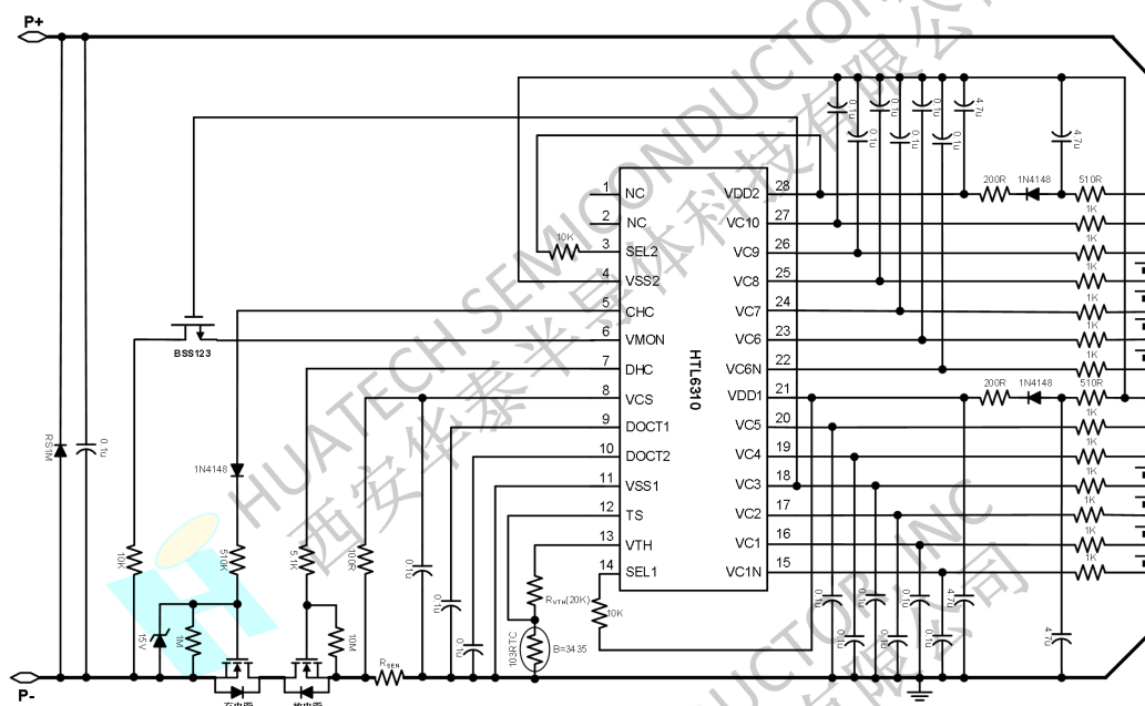
图 4 8 节电池包的 N 型充电管和 N 型放电管的同口典型应用电路图
