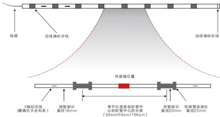
柔性测斜仪产品形态
