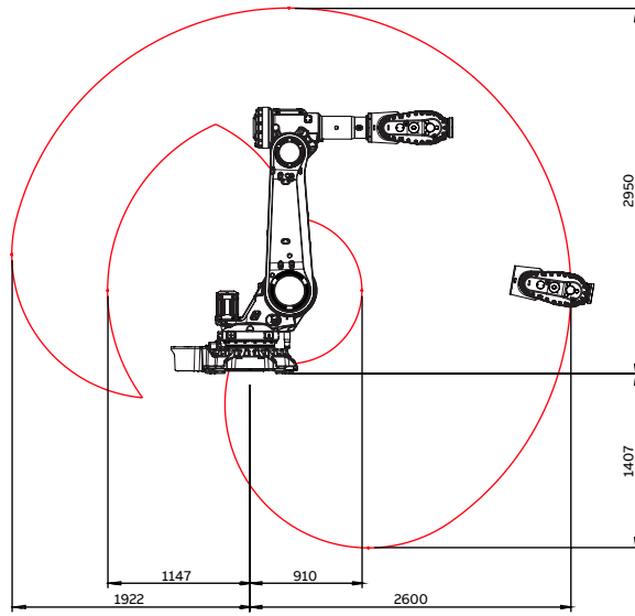
IRB 5720-180/2.6 工作范围
