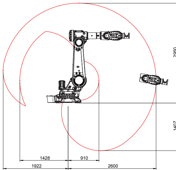
IRB 5720-155/2.6 LID 工作范围
