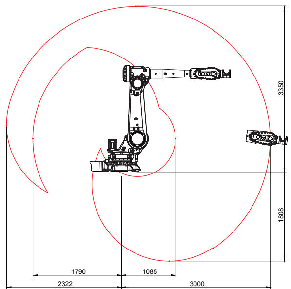
IRB 5720-90/3.0 LID 工作范围
