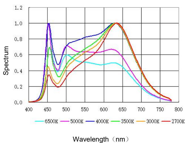
相对光谱分布曲线图 Relative Spectral Distribution
