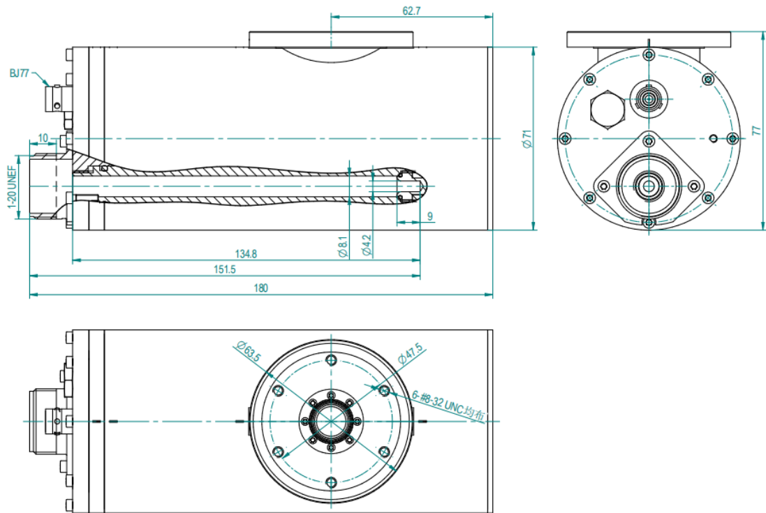
外形图
