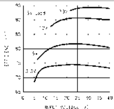
图 7-3. Efficiency
