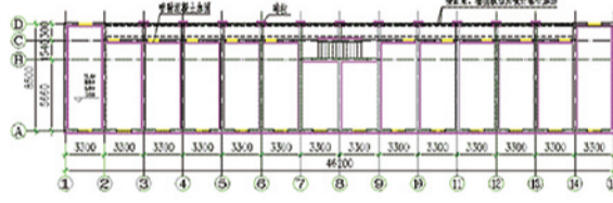
图5 加固平面布置图
