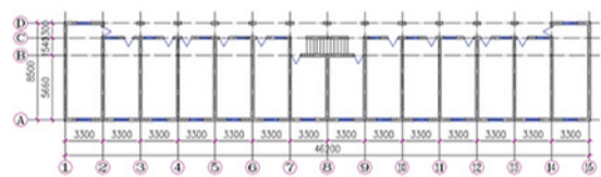
图1 房屋结构平面图
