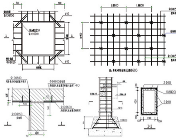
图4 加固设计详图
