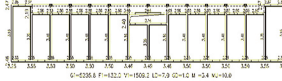
图6 一层抗震验算结果(抗力与效应之比)
