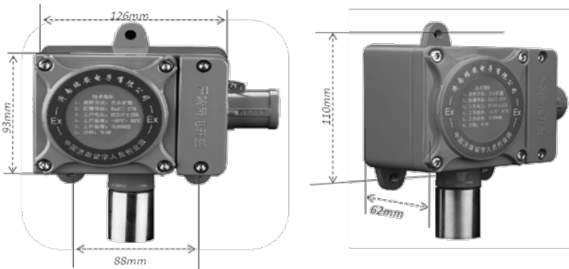
图 5-1 探测器尺寸
