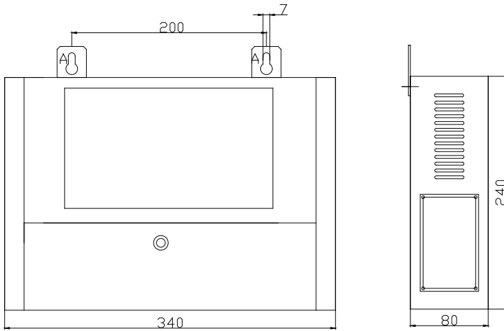
图 4-1 : RBK-6000-6 机箱尺寸（单位：mm）
