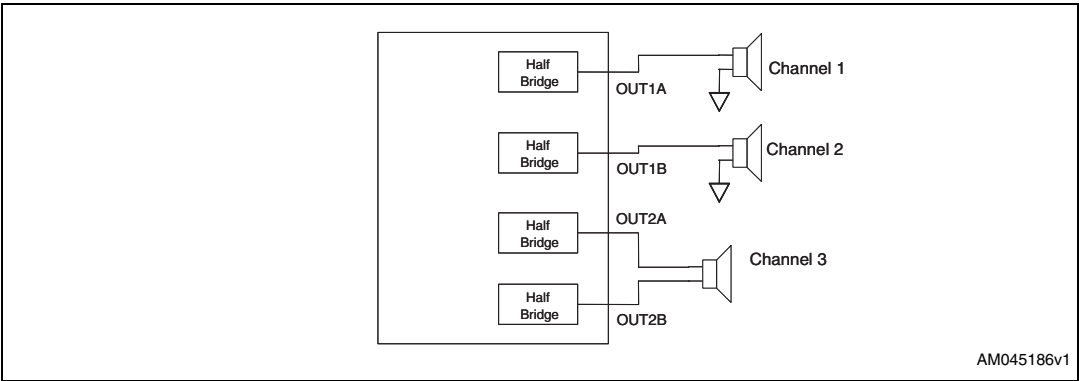
Figure 25. OCFG = 10
