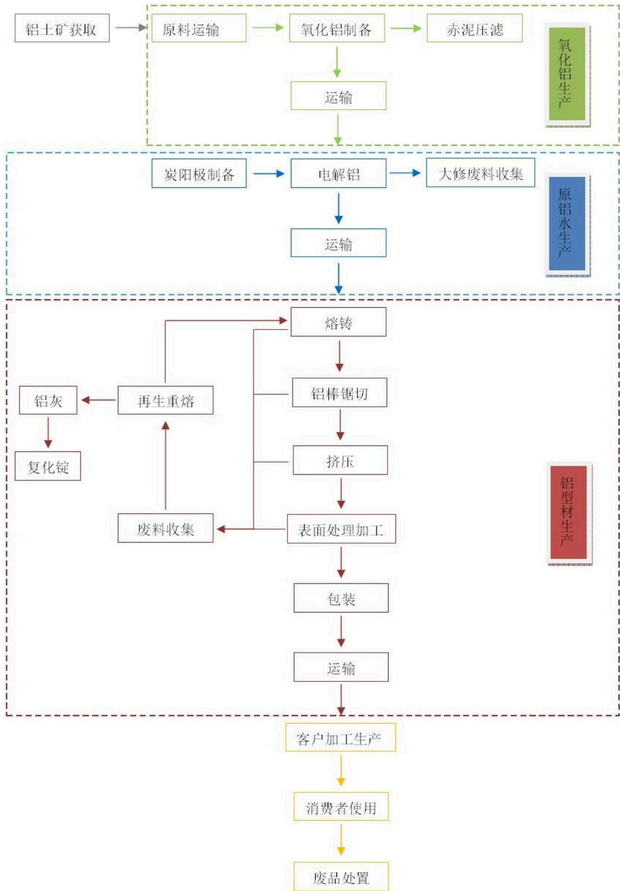
图1 铝型材生命周期评价范围（全产业链）
