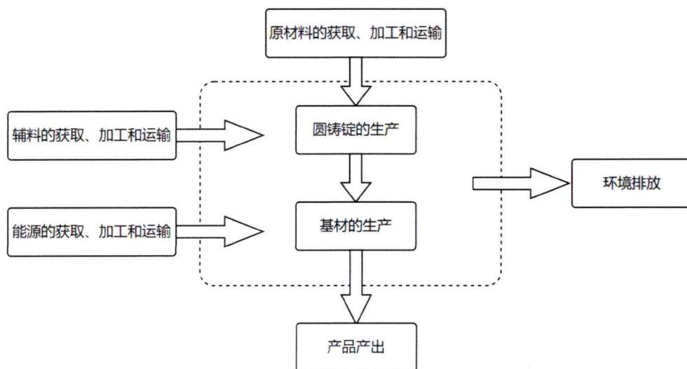
图3-3 1吨铝合金建筑型材（基材型材）产品LCA研究边界
