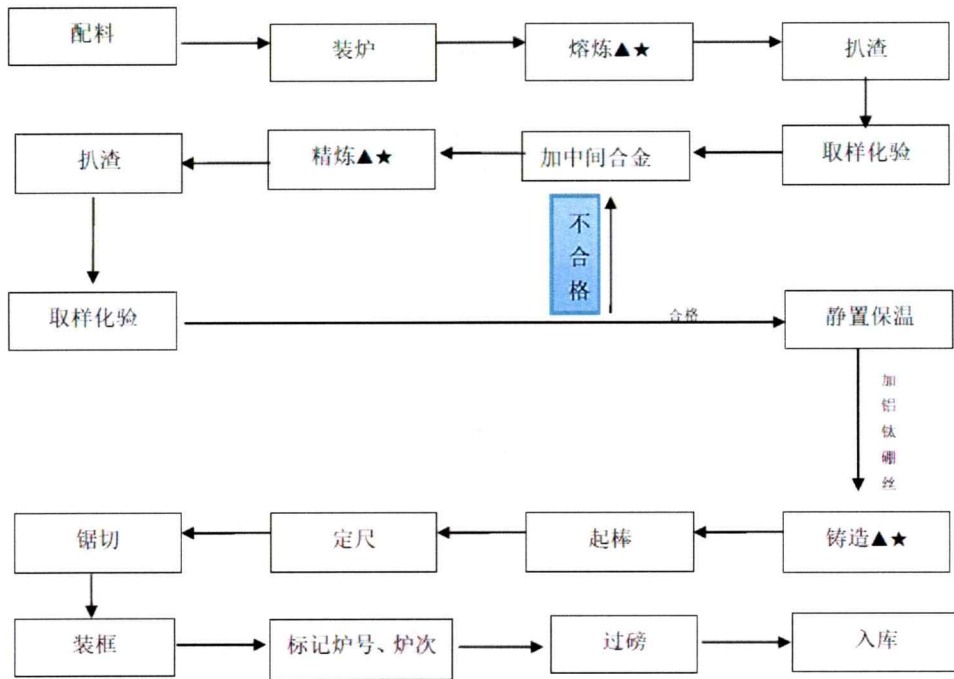
图3-1 圆铸锭生产工艺流程图
