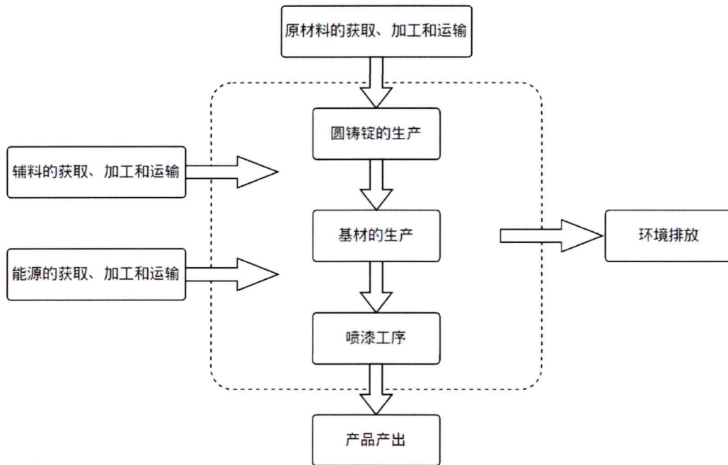
图3-4 1吨铝合金建筑型材（喷漆型材）产品LCA研究边界
