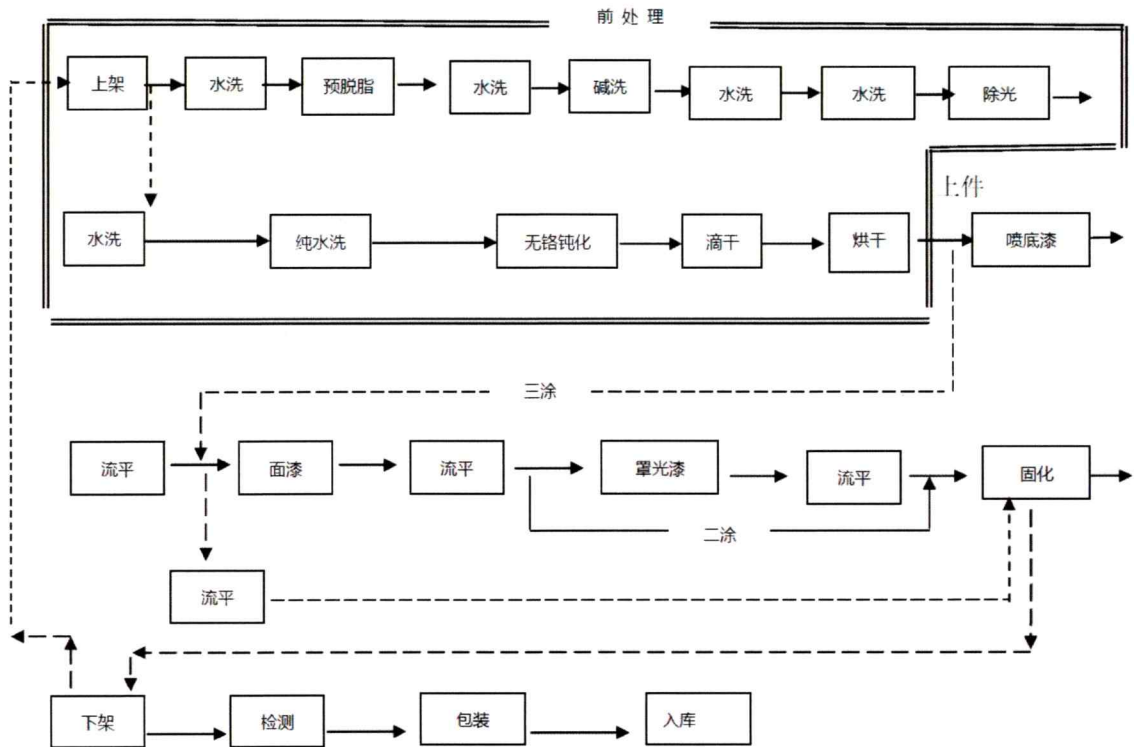
图3-3 喷漆工艺流程
