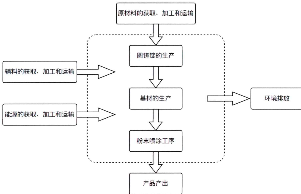
图3-3 1吨铝合金建筑型材（喷粉型材）产品LCA研究边界
