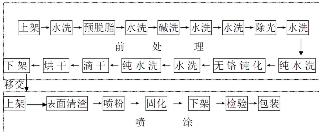
图3-3 粉末喷涂工艺流程
