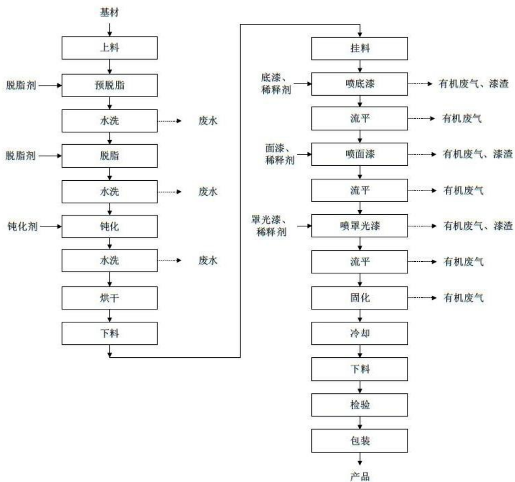
图 4 喷漆生产线生产工艺流程图
