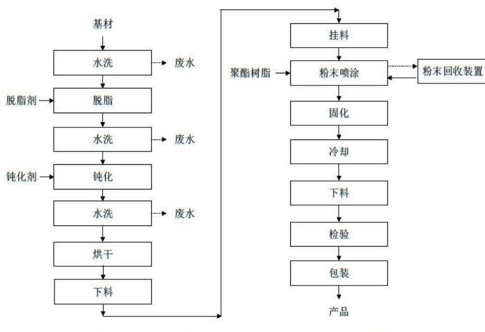
图 5 喷粉生产线生产工艺流程
