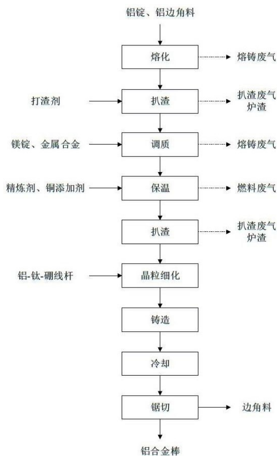
图 1 熔铸车间生产工艺流程图
