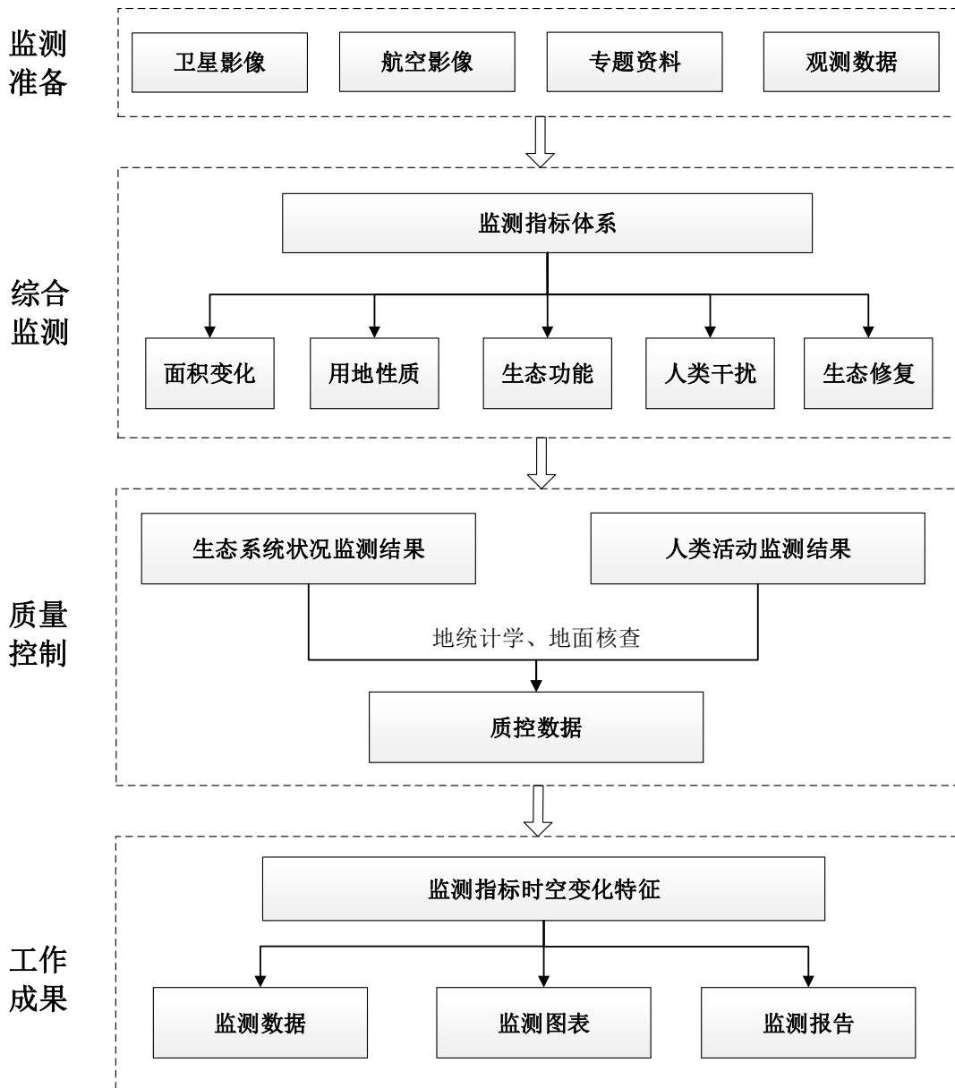
图 1 生态保护红线生态状况监测技术流程图
