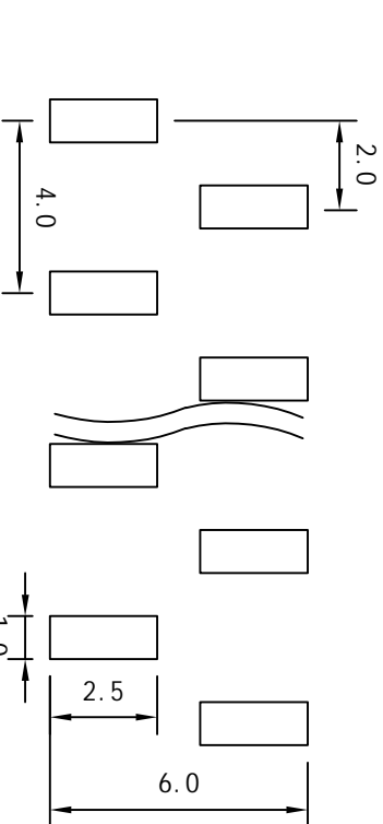
P.C.B LAYOUT
