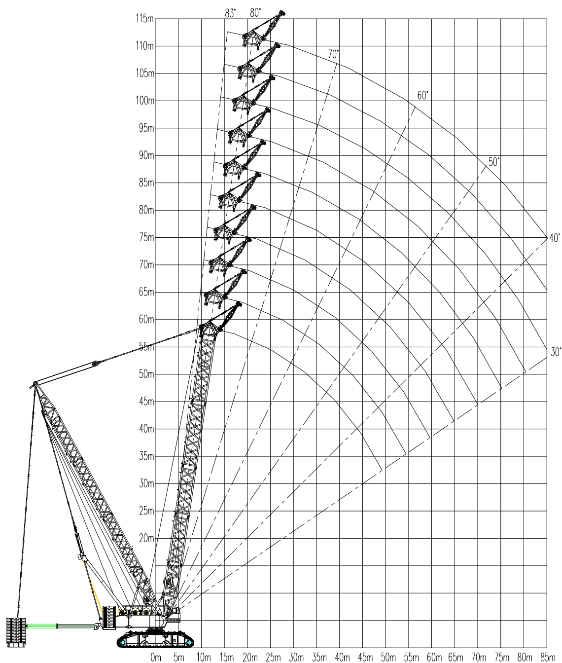
图 3-1 XGC28000 SLB 超起工况起轻型主臂作业范围图
