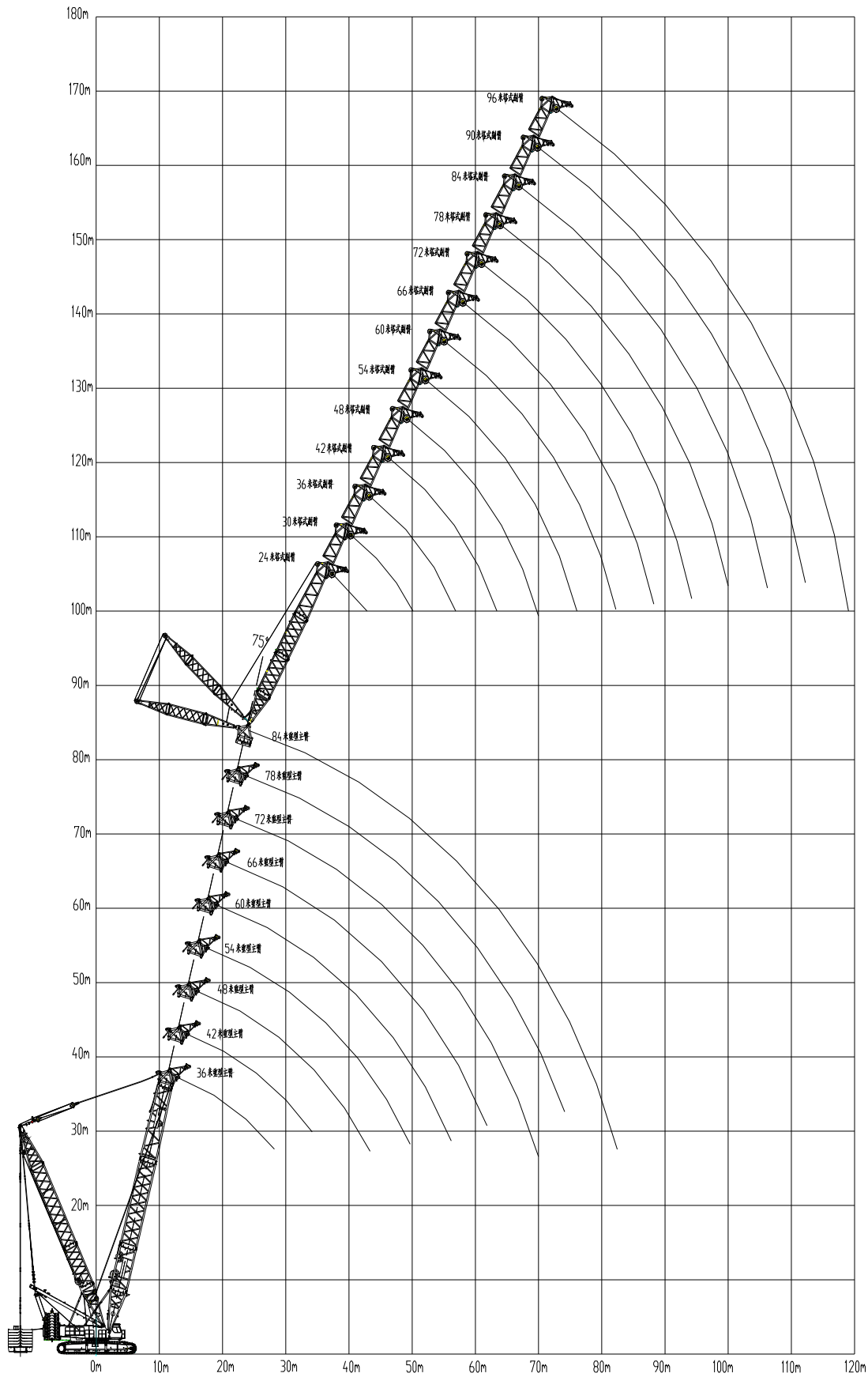
图 4-2 XGC28000 超起工况塔式副臂作业范围图主臂仰角 75°
