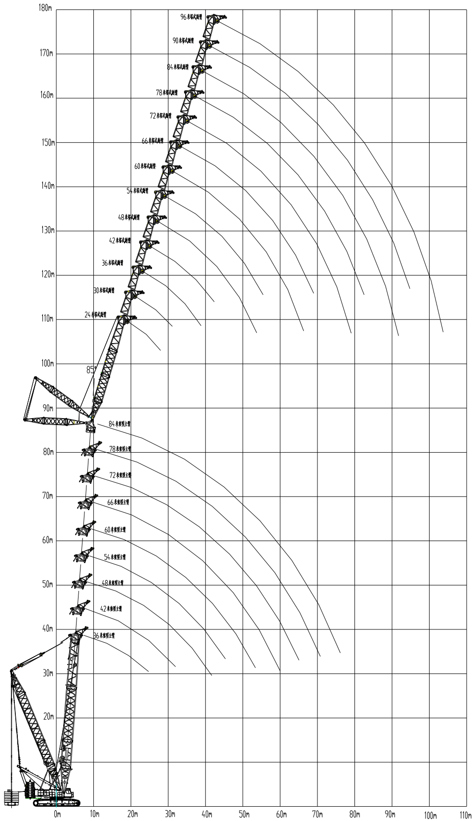
图 4-1 XGC28000 超起工况塔式副臂作业范围图主臂仰角 85°
