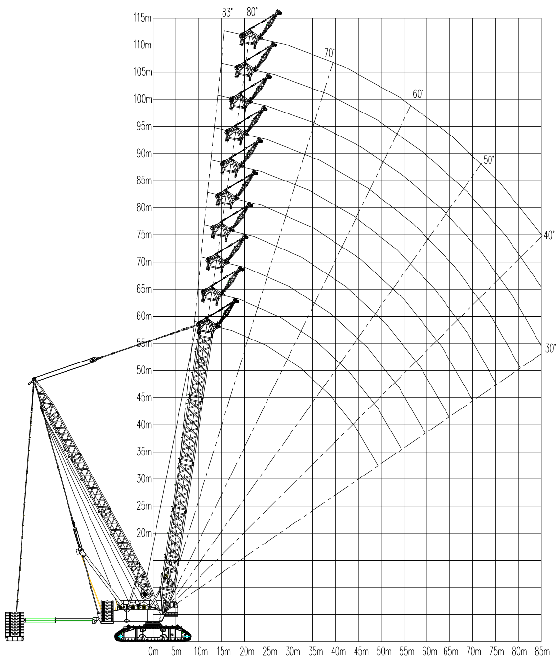
图 2-1 XGC28000 SHB 超起工况重型主臂作业范围图
