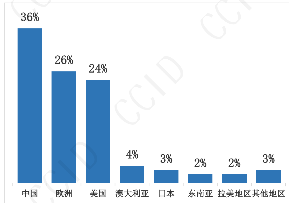
2022年全球新增投运新型储能项目的地区分布 (MW%) 数据来源: CNESA
