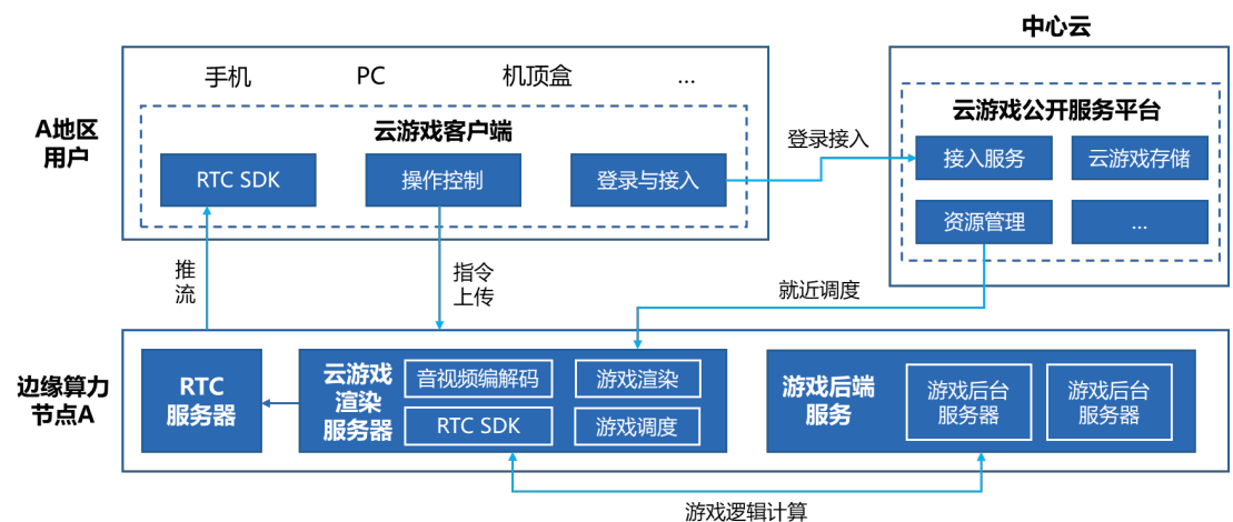
图 4.5 基于边缘算力的云游戏系统架构
