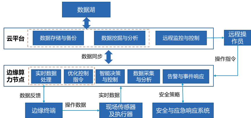
图 4.4 数字化变电站典型应用架构图
