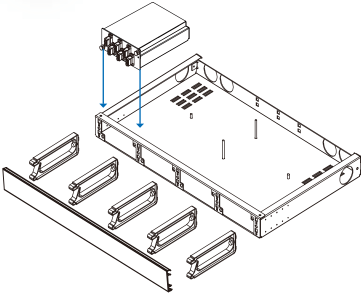
高密度光纤收容箱 ( p/n: FL-FR0104BK ) 可同时安装四个预端接光纤模组
