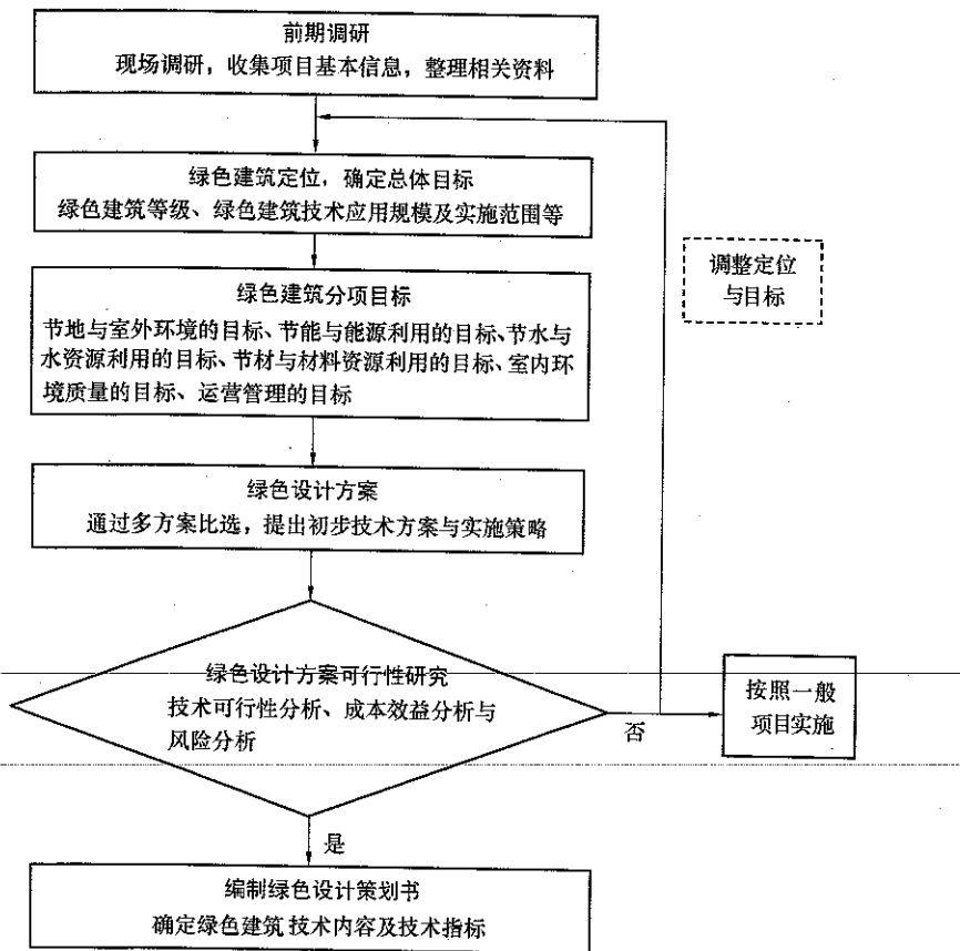
图 1 绿色设计策划流程图
