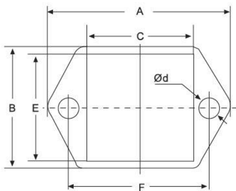
H3A开孔底座
