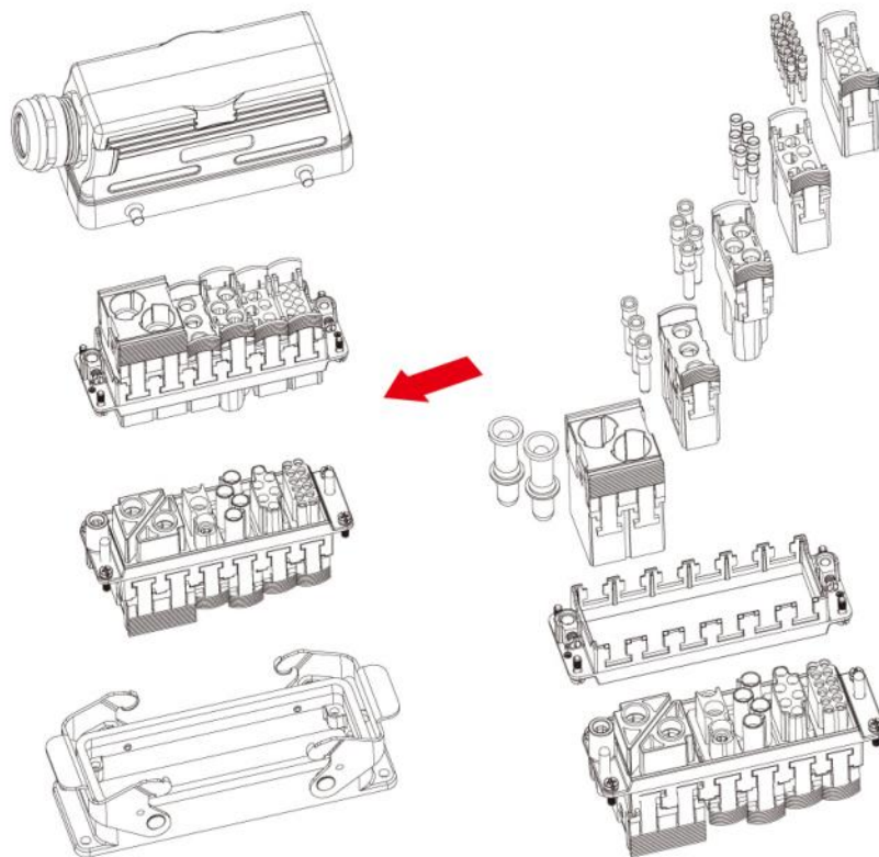
HMN组合模块安装示意图
