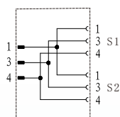
3针公插转2个3针母插 电路原理图
