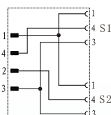
4针公插转2个3针母插 电路原理图
