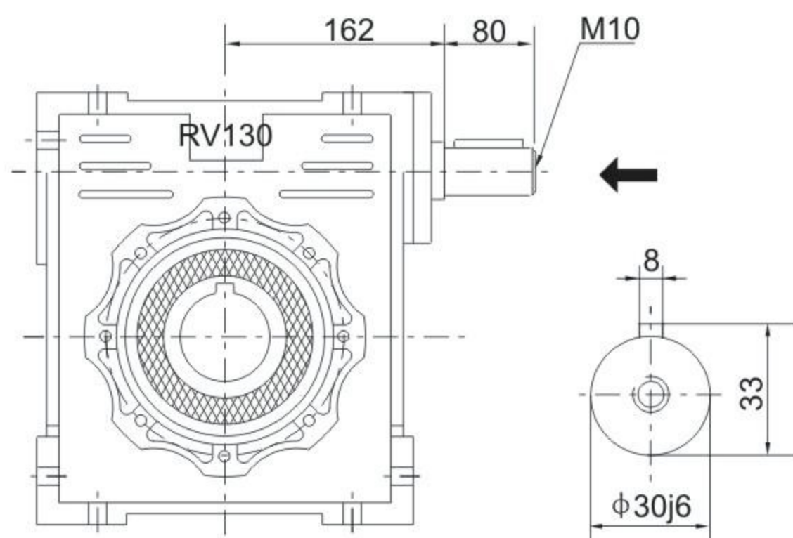
NRV130
