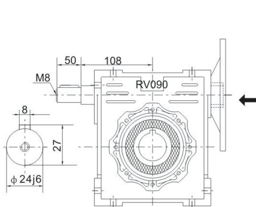
NMRV090.....E
