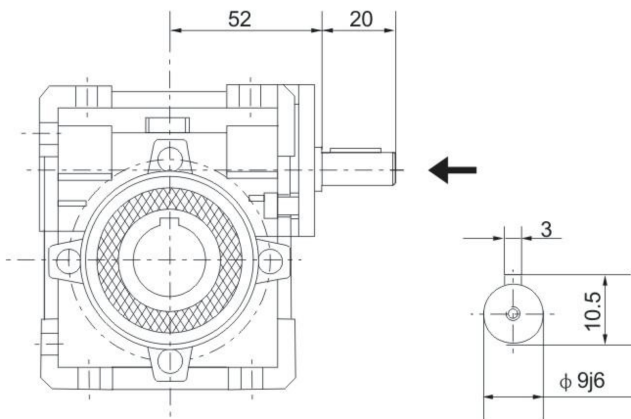
NRV030
