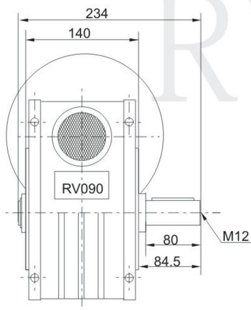
NMRV090.....DZ
