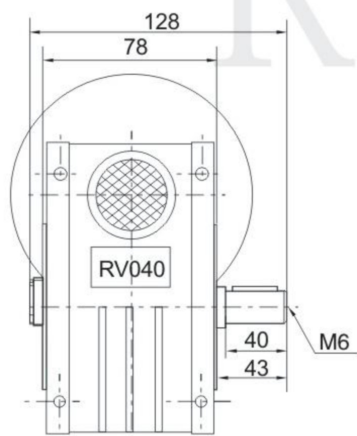
NMRV040.....DZ
