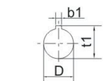
蜗杆输入孔
