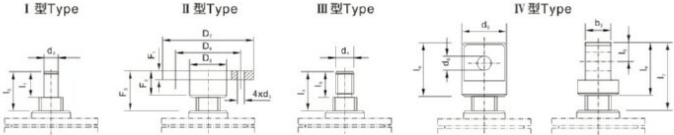
图1 I 型结构型式 Type I structural mode
