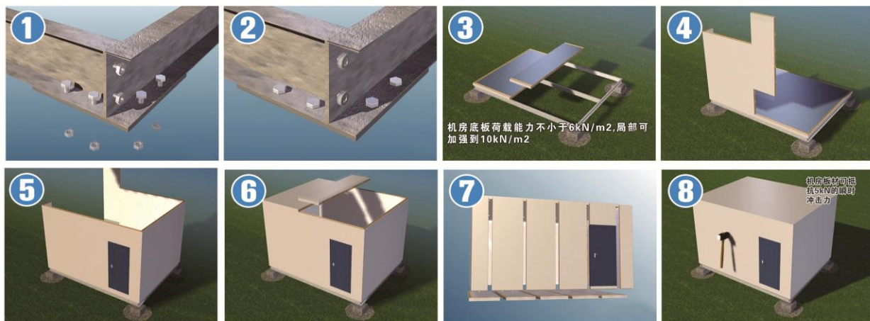
拼装式通信 机房保温结构板
