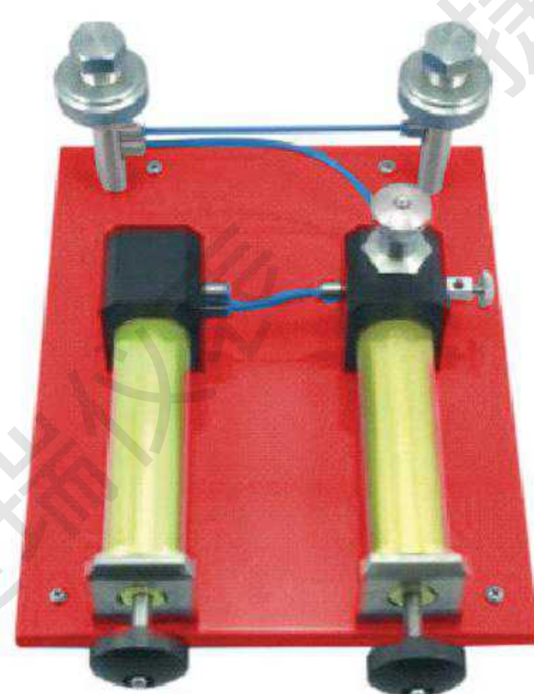
YLJ1009型低压气体压力源
