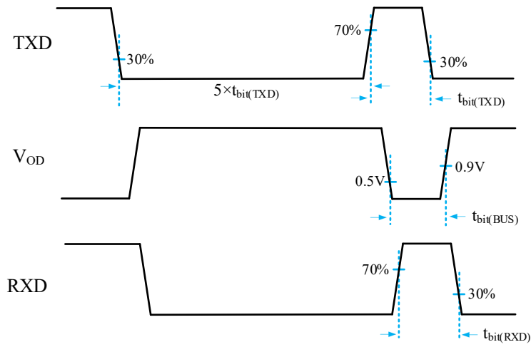
图 8 t_{\text{bit}} 延时示意图
