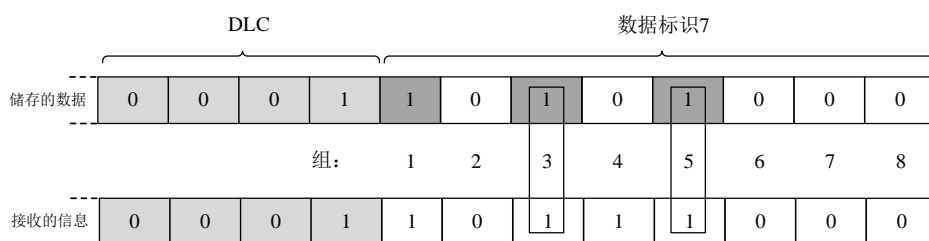
图 7 在选择性唤醒帧中评估数据字段
