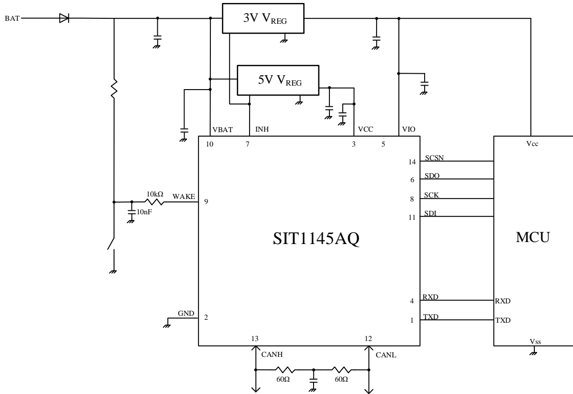
图 16 典型应用示意图
