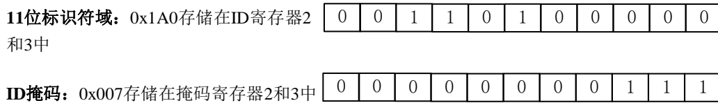
图6 评估选择性唤醒帧中的 ID 字段
