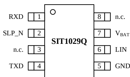
图 2 SIT1029Q 引脚分布图
