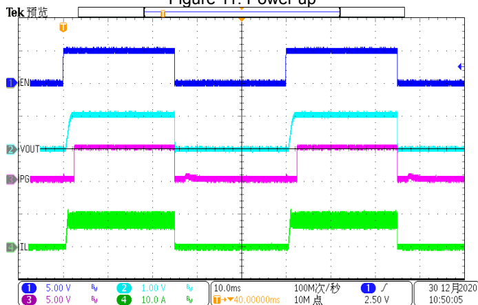
Figure 13. EN toggle (Iload=8A)
