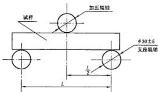
图 12 抗折强度试验机示意图
