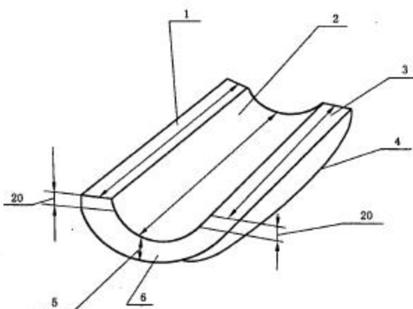
图1 板、块尺寸测量方法示意图
