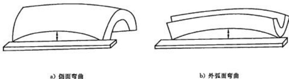
图8 管壳与弧形板弯曲测量方法示意图
