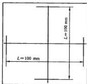
图 13 匀温灼烧线收缩率测点布置示意图
