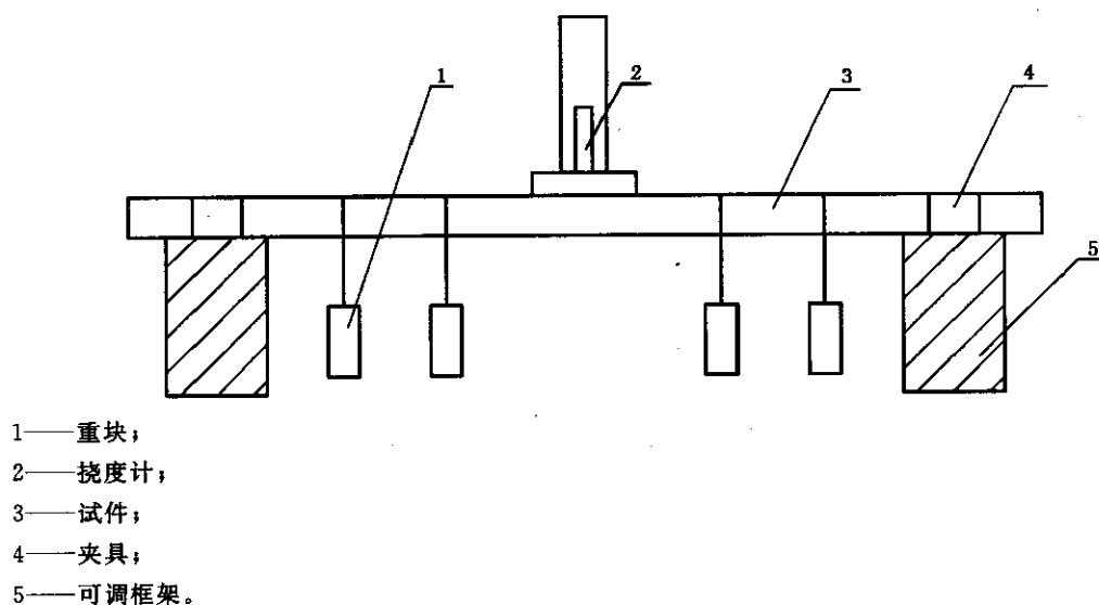
图 6 卷轴挠度测量装置示意图
