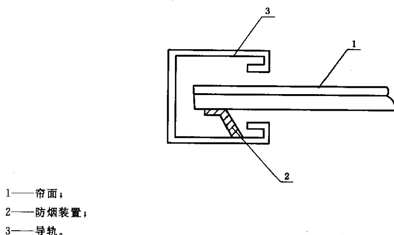
图3 导轨防火装置示意图
