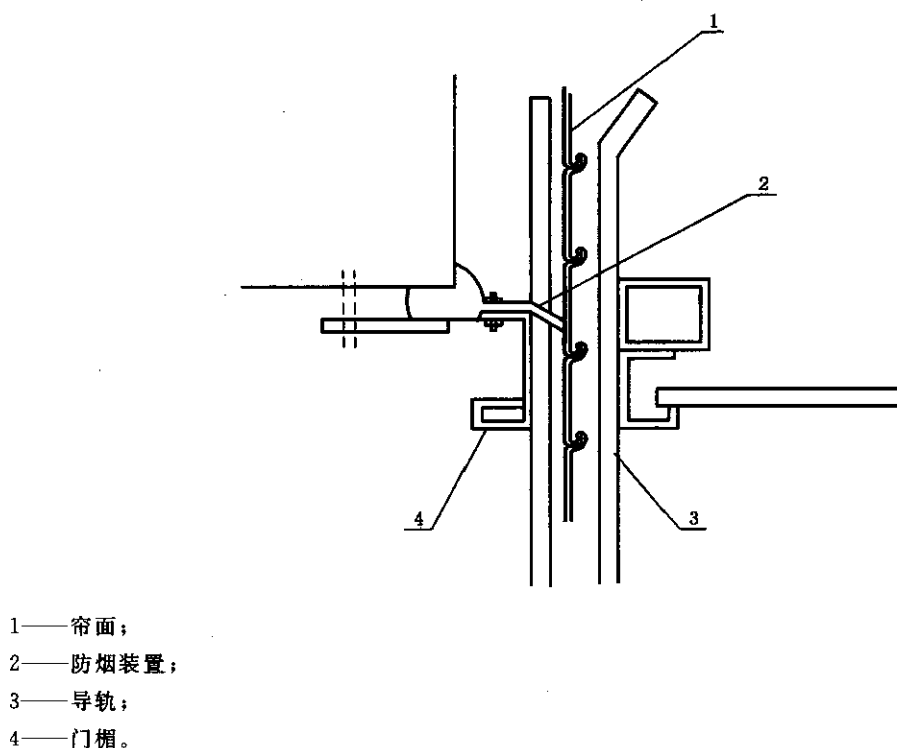
图4 门楣防火装置示意图
