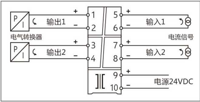
2 入 2 出, 直流信号输出隔离器---端子接线图
