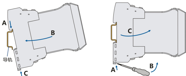
安装在导轨上示意图
