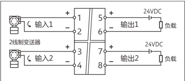
2 入 2 出，二线回路配电隔离器—端子接线图
