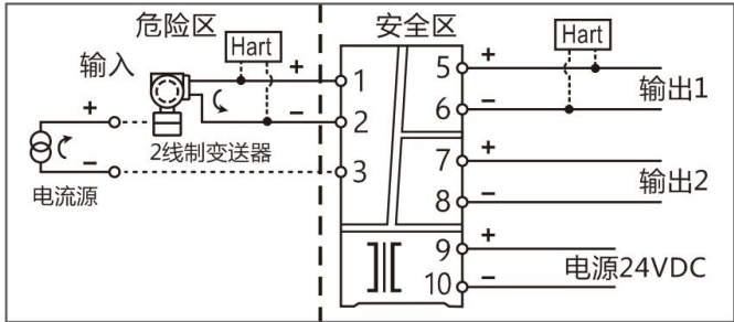
1 入 2 出、1 入 1 出，配电或电流输入安全栅(HART 通过)---端子接线图 * 注：1 入 2 出、1 入 1 出产品，HART 信号通过均从端子 5/6 接入。 1 入 1 出的产品无输出 2，端子 7/8 不用。
