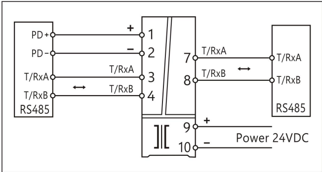
RS485通信隔离器（12V配电，RS485转RS485）---端子接线图 注：无配电功能时，接线时端子1/2不用。
