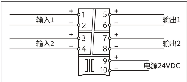
2入2出，直流信号输入隔离器 (电流或电压信号输入/电流或电压信号输出)——端子接线图
