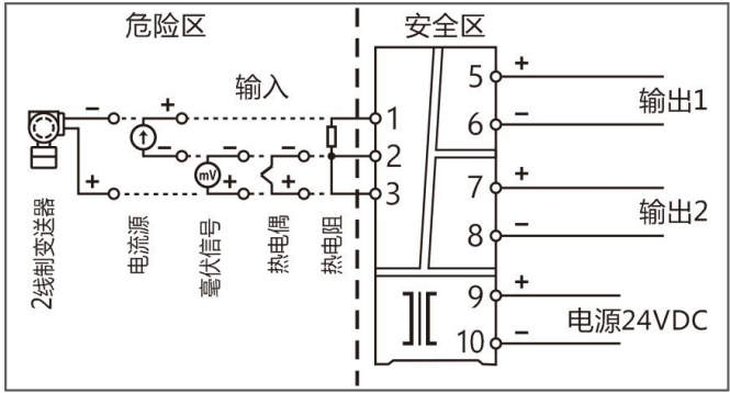
1 入 2 出, 通用信号输入隔离器—端子接线图
