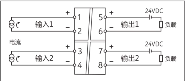
2 入 2 出，二线回路电流信号隔离器—端子接线图
