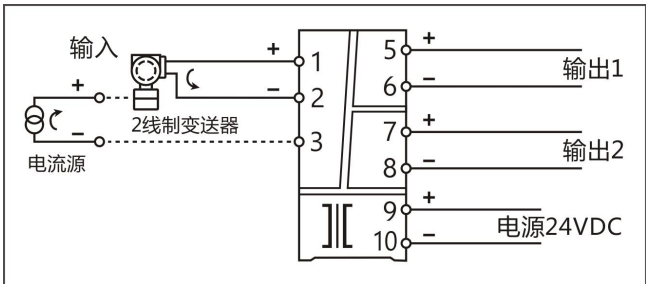
1入2出，直流信号输入隔离器(4~20mA 输入/直流信号输出)——端子接线图
