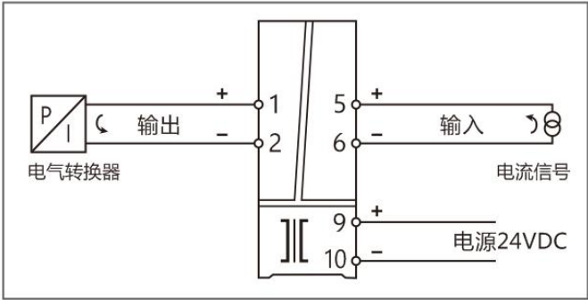
1 入 1 出, 直流信号输出隔离器---端子接线图
