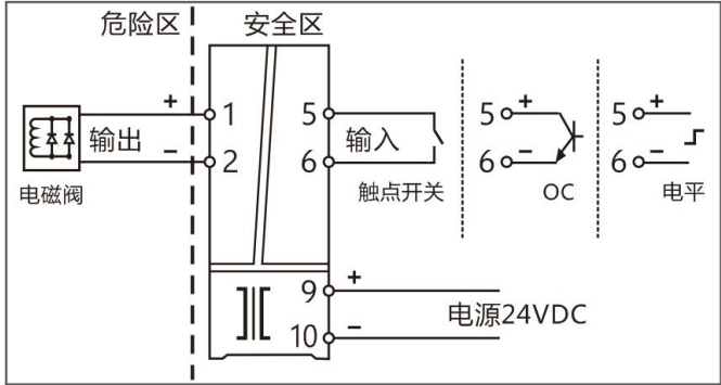
1 入 1 出，开关量输出安全栅---端子接线图
