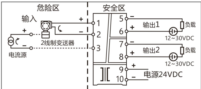
1 入 2 出、1 入 1 出，配电或电流输入安全栅(输出外供电)---端子接线图 * 注：1 入 1 出产品无输出 2，端子 7/8 不用。
