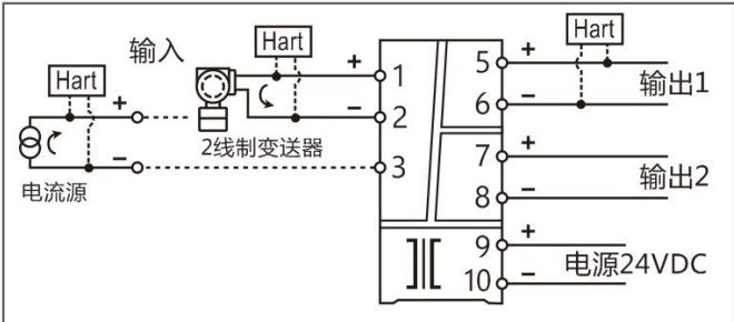
1 入 2 出、1 入 1 出，配电或电流输入隔离器(HART 通过)---端子接线图 * 注：1 入 1 出的产品无输出 2，端子 7/8 不用。
