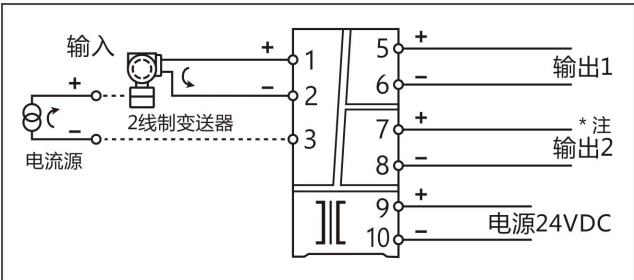
1 入 2 出、1 入 1 出，配电或电流输入隔离器---端子接线图 * 注：1 入 1 出产品无输出 2，端子 7/8 不用。
