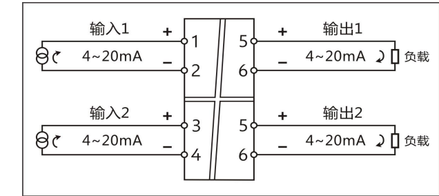
2 入 2 出, 无源隔离器—端子接线图
