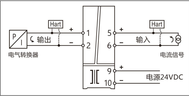
1 入 1 出, 直流信号输出隔离器(支持 HART 通过)---端子接线图
