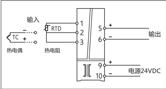
1 入 1 出，热电阻或热电偶输入隔离器—端子接线图
