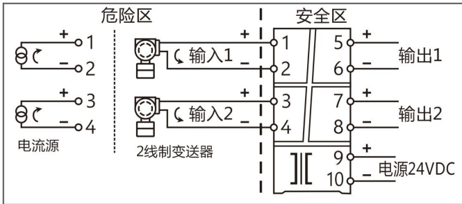
2 入 2 出，配电或电流输入安全栅---端子接线图
