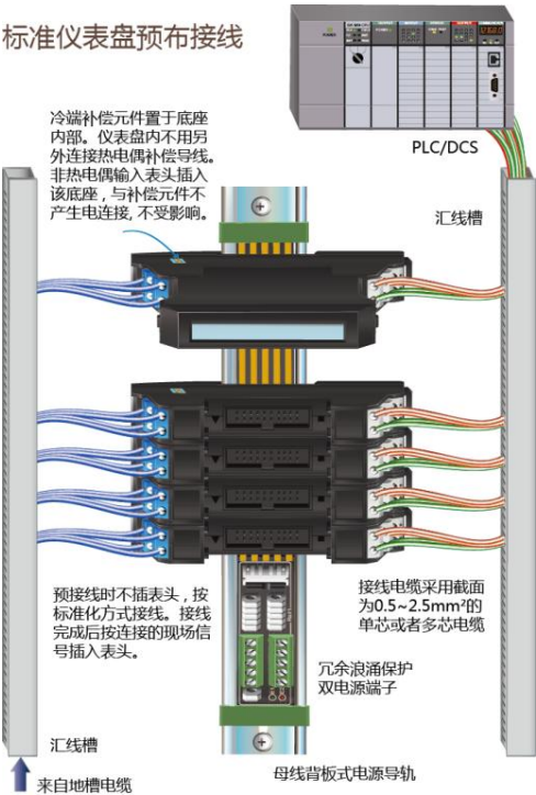
图 C DS(DSA)预接线示意图
