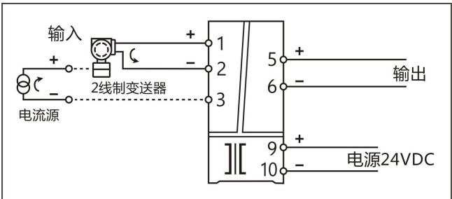
1入1出，直流信号输入隔离器(4~20mA 输入/直流信号输出)——端子接线图
