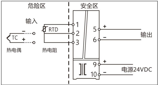
1入1出，热电阻或热电偶输入安全栅—端子接线图
