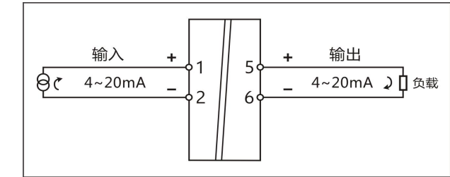
1 入 1 出, 无源隔离器—端子接线图
