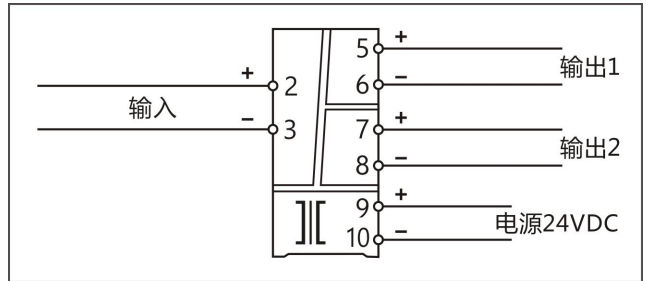
1入2出，直流信号输入隔离器 (电流或电压信号输入/电流或电压信号输出)——端子接线图
