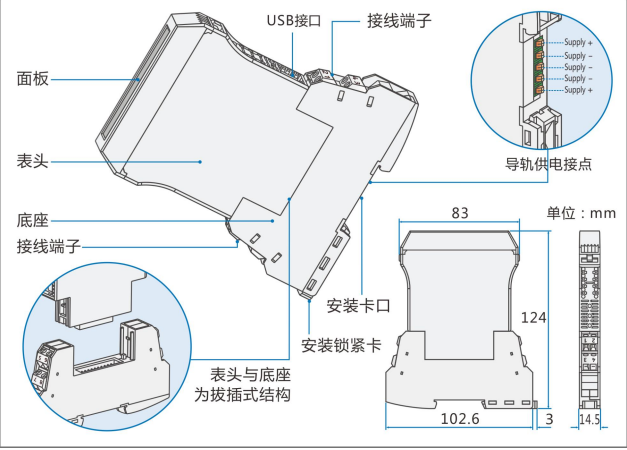
图 A DS(DSA)外形结构/尺寸
