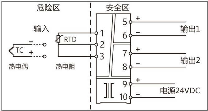
1入2出，热电阻或热电偶输入安全栅—端子接线图
