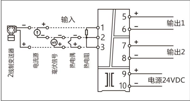
1 入 2 出，通用信号输入隔离器—端子接线图
