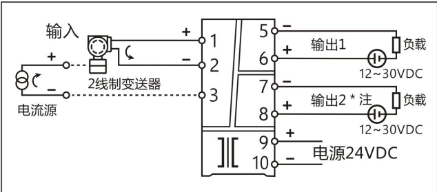
1 入 2 出、1 入 1 出，配电或电流输入隔离器(输出外供电)---端子接线图 * 注：1 入 1 出产品无输出 2，端子 7/8 不用。
