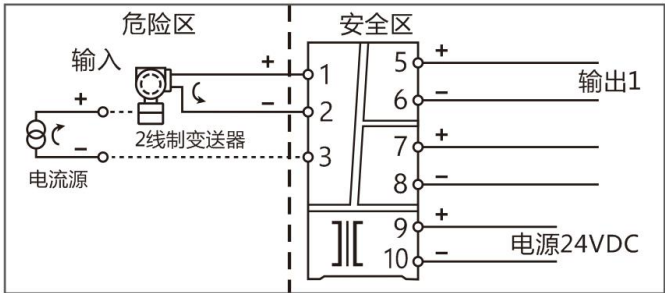
1 入 2 出、1 入 1 出，配电或电流输入安全栅---端子接线图 * 注：1 入 1 出产品无输出 2，端子 7/8 不用。
