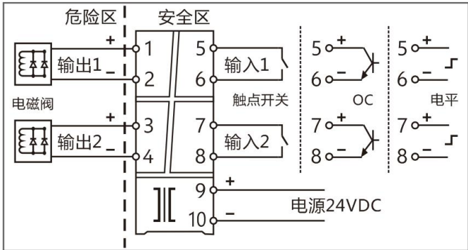
2入2出，开关量输出安全栅---端子接线图
