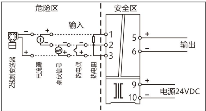
1 入 1 出, 通用信号输入隔离器—端子接线图
