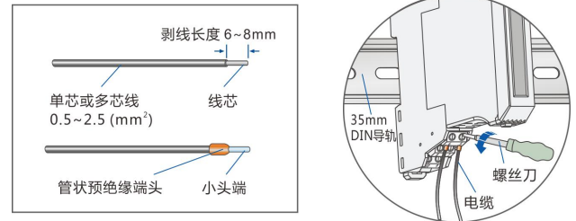
螺丝连接示意图
