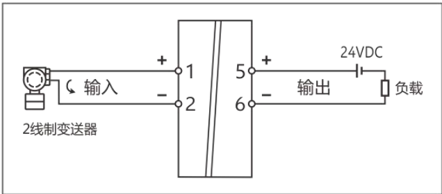
1 入 1 出，二线回路配电隔离器—端子接线图
