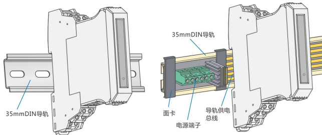
图 A 标准导轨卡式安装示意图
