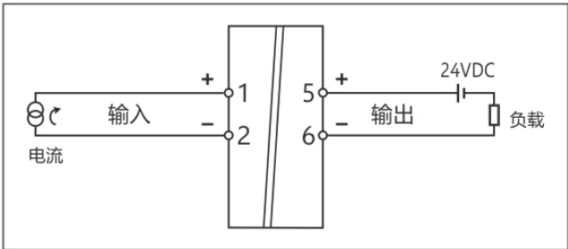
1 入 1 出，二线回路电流信号隔离器—端子接线图
