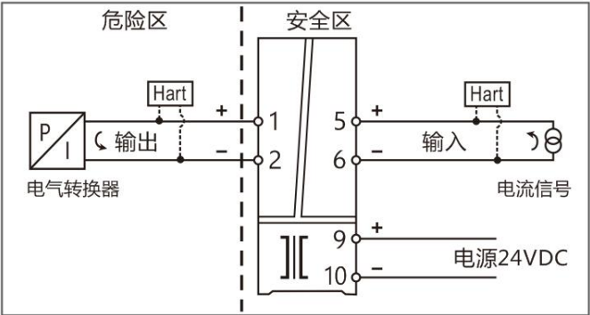
1 入 1 出, 直流信号输出安全栅(支持 HART 通过)---端子接线图
