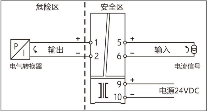
1 入 1 出, 直流信号输出安全栅---端子接线图
