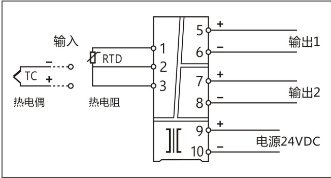
1 入 2 出，热电阻或热电偶输入隔离器—端子接线图
