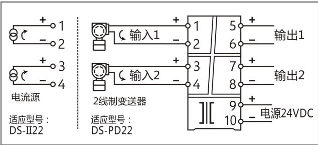
2 入 2 出，配电或电流输入隔离器---端子接线图
