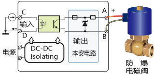
本安和三隔离配置原理图
