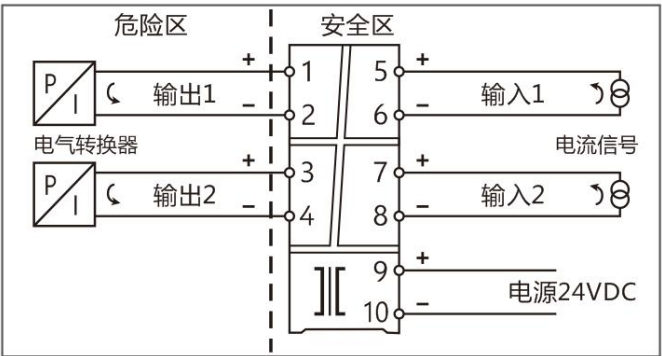
2 入 2 出, 直流信号输出安全栅---端子接线图
