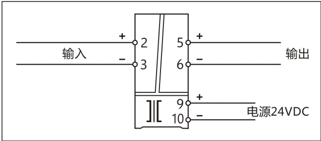
1入1出，直流信号输入隔离器 (电流或电压信号输入/电流或电压信号输出)——端子接线图
