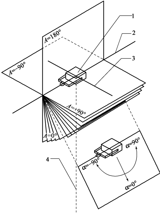
图 1 A- \alpha 测量几何示意图
