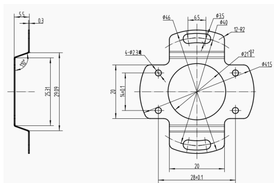
MP4409-002A-40 (C型——安装孔d40) 板弹簧机械尺寸图
