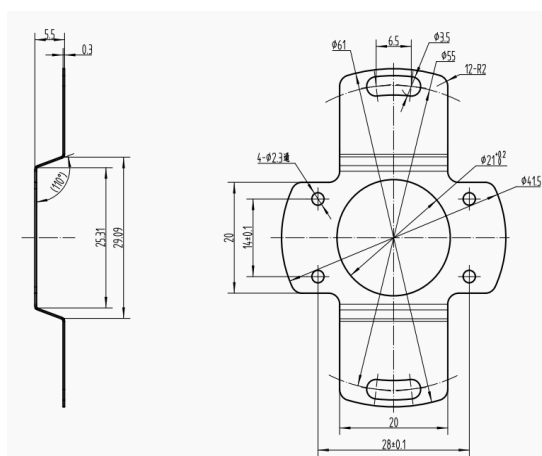
MP4409-001A-55 (D型——安装孔d55) 板弹簧机械尺寸图
