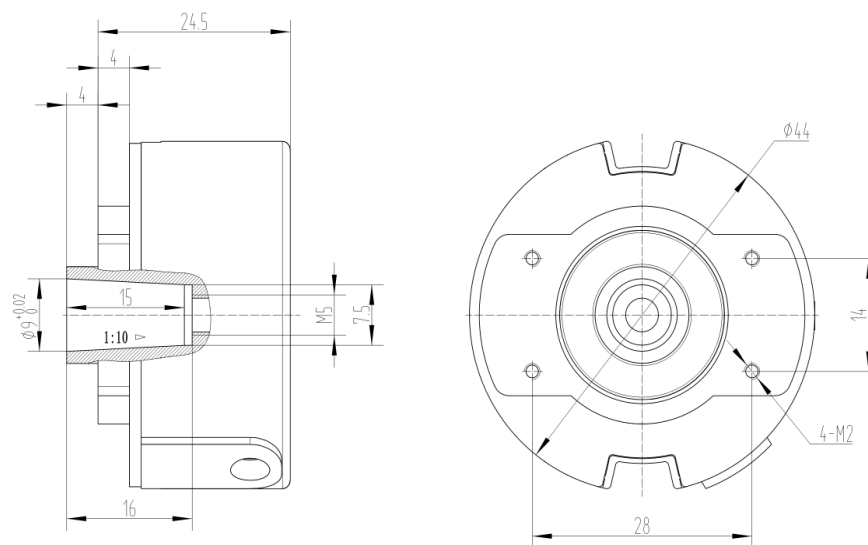
UZ4409机械尺寸图
