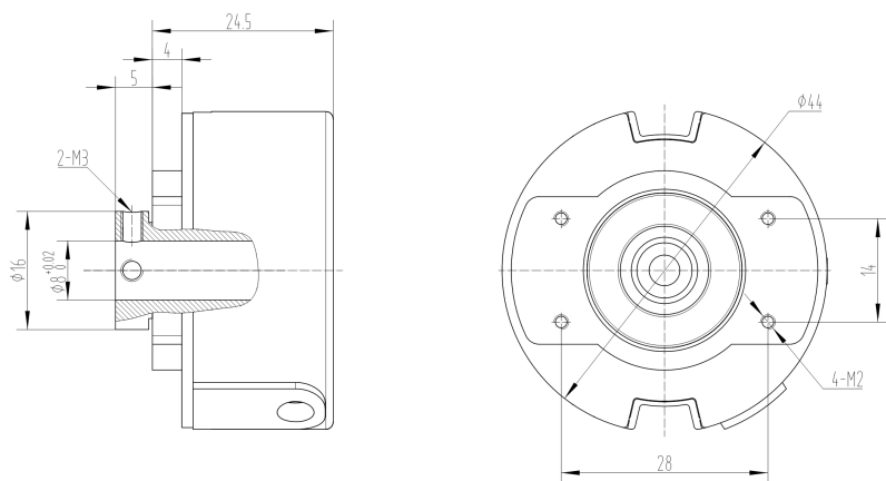
UZ4408机械尺寸图
