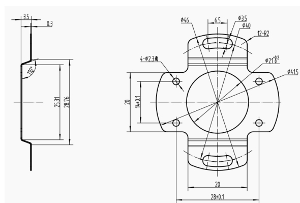
MP4409-003A-40 (CL型——安装孔d40) 板弹簧机械尺寸图
