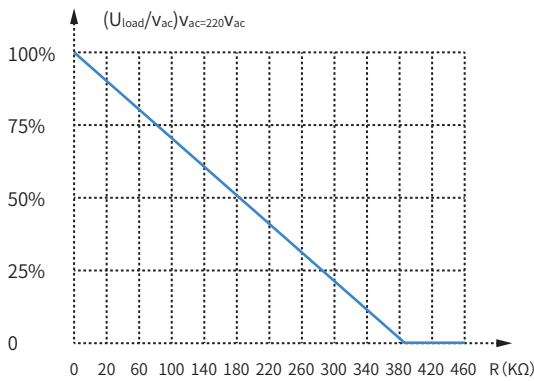
输出vs.调节电位器470 (kΩ)
