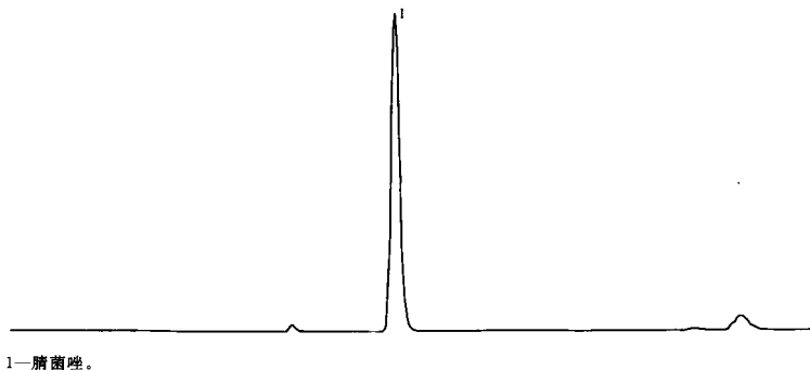
图2 腈菌唑原药的高效液相色谱图
