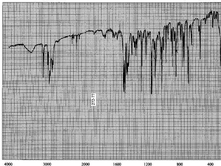
图 1 腈菌唑标样红外光谱图
