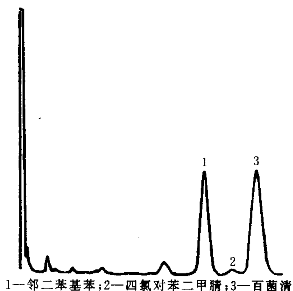
图 1 百菌清烟粉粒剂气相色谱图
