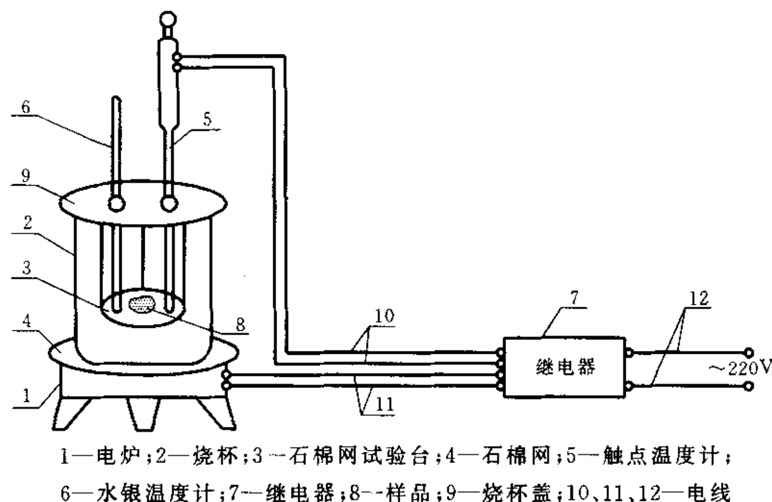
图3 自燃温度测定仪
