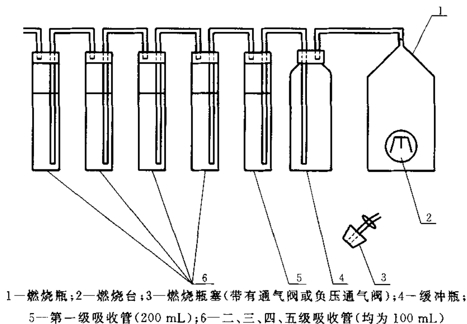
图 4 成烟及收集装置图
