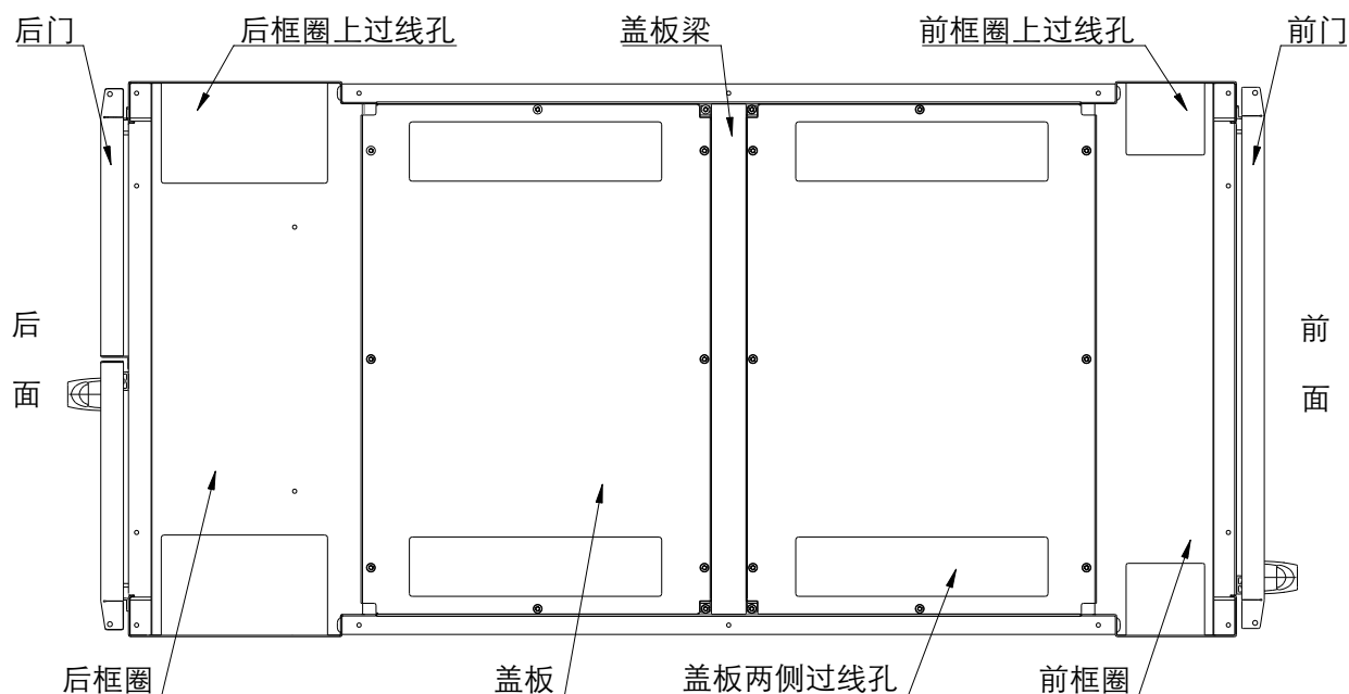
图 24: 机柜顶部过线孔位置示意图
