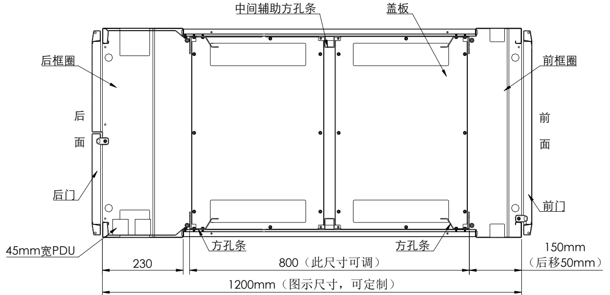
图 18：机柜内部方孔条移位安装位置示意图
