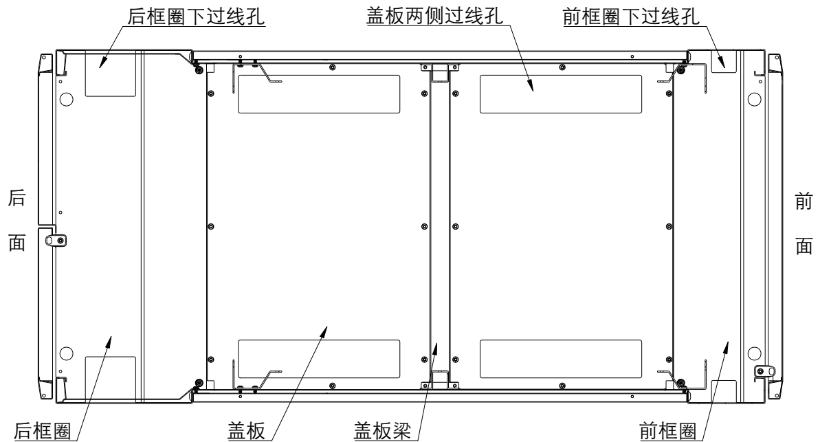
图 25: 机柜底部过线孔位置示意图
