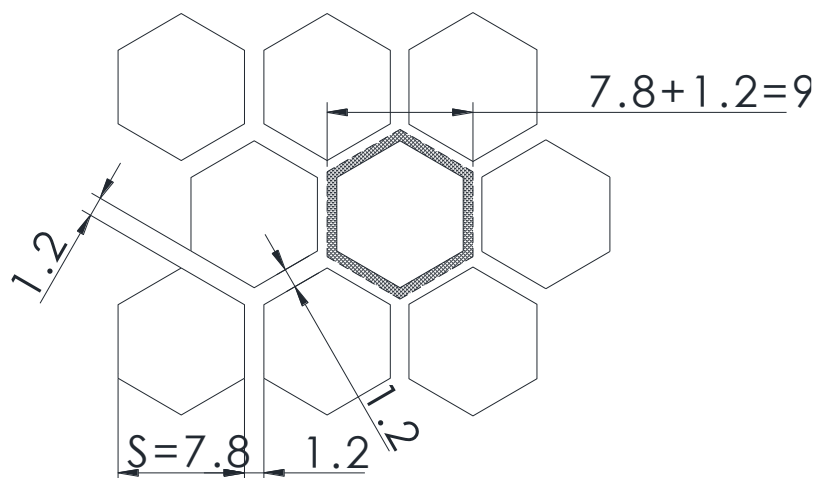
图 11: 机柜门板上六角孔示意图
