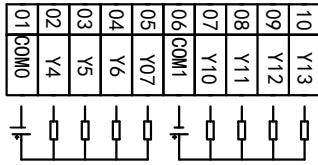
4.3寸一体机MC_20MT_6MT_i430A_FX_A接线图
