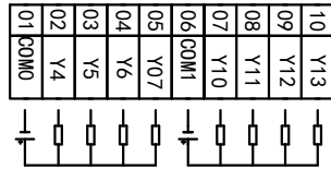
4.3寸一体机MC_20MT_6MT_430A_FX_A接线图 V2
