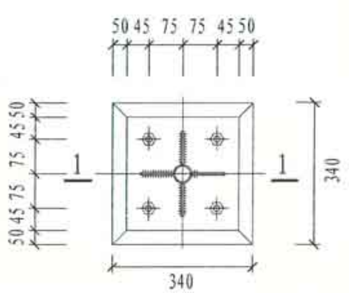
④ 屋面旗杆座俯视图
