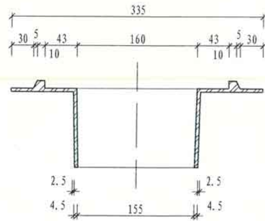
③ 环形筒剖面图
