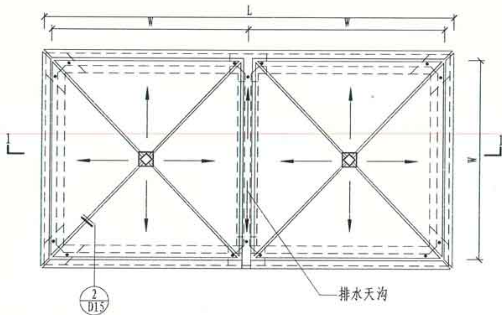
隐框四面锥采光顶平面示意图
