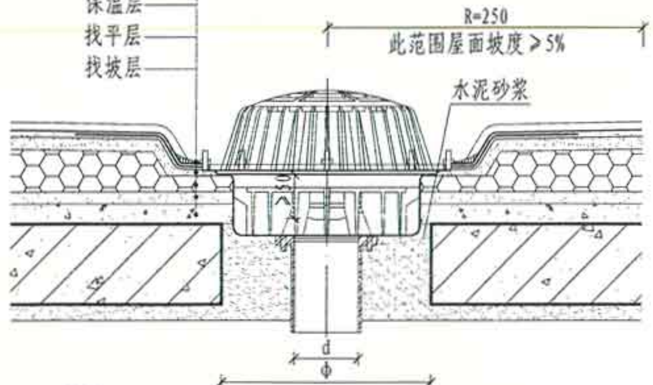
① 虹吸式雨水斗在屋面 (天沟) 板上安装 (YG50、75、80、100A型)
