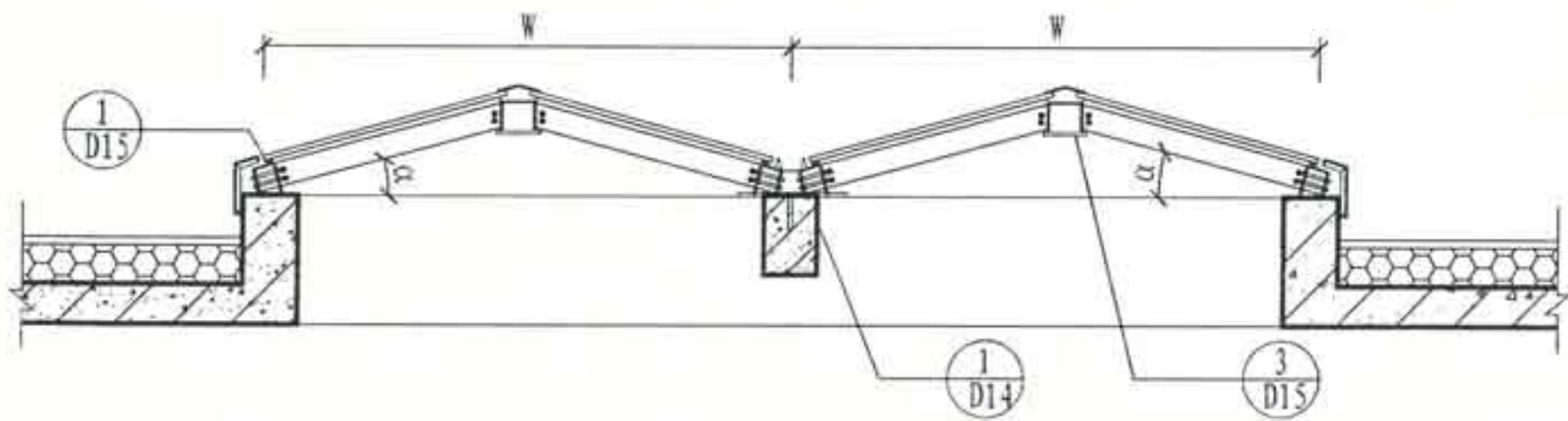
1-1剖面图
