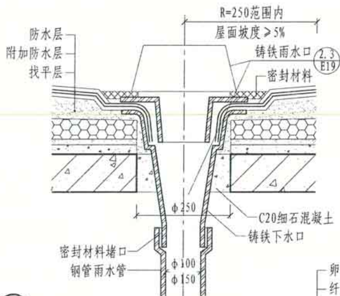
⑤ 内排水铸铁雨水口
