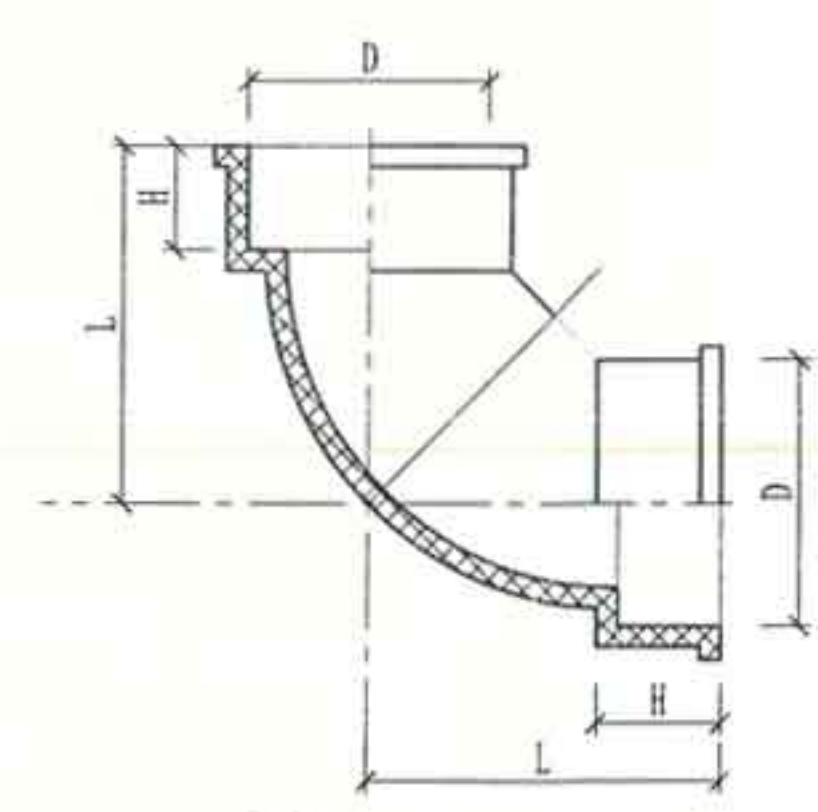
⑧ UPVC90° 弯头
