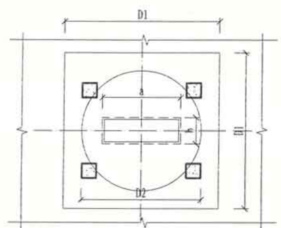
B-B自力式风帽平面图
