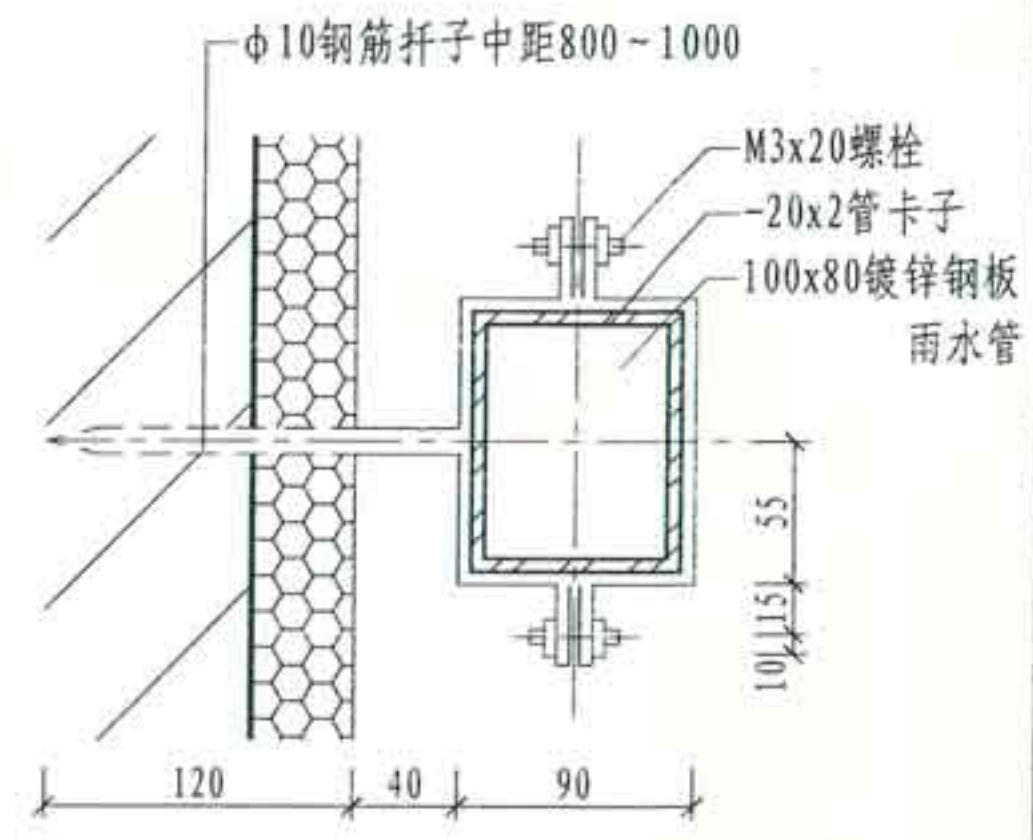
⑥ 方雨水管及卡子
