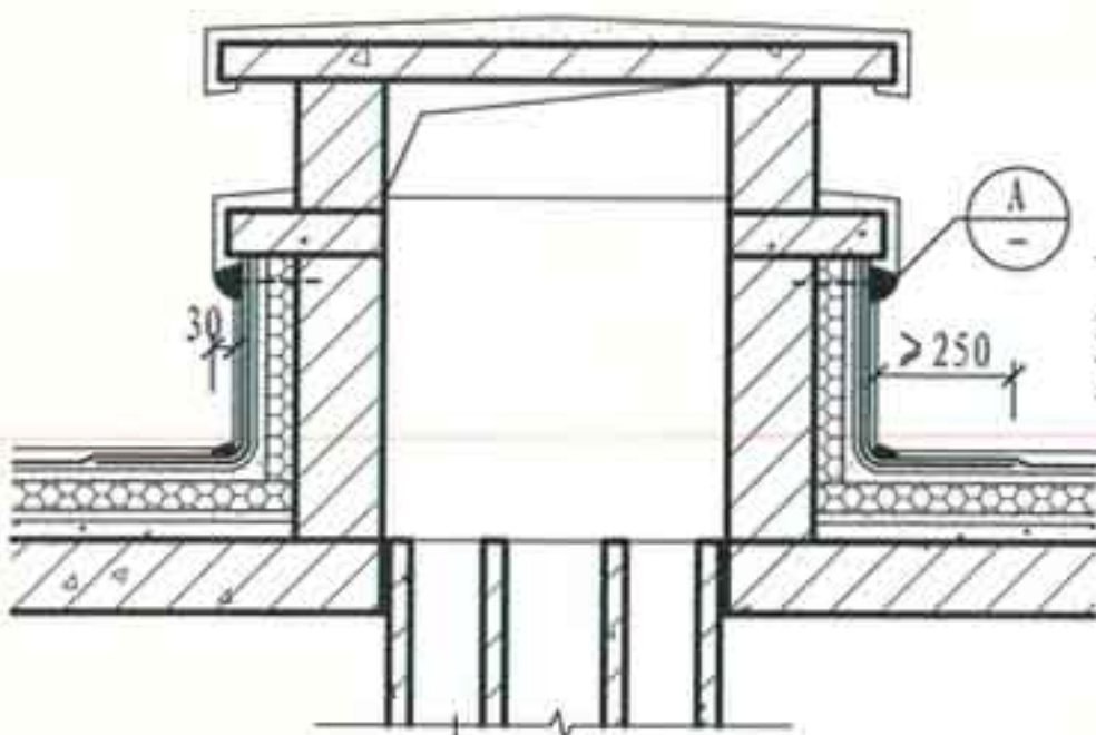
2-2 当采用钢筋混凝土预制通风道时，通风道伸入楼板内
