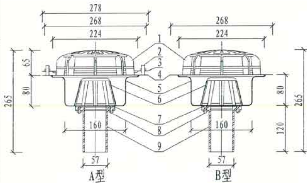
① YG50型虹吸式雨水斗
