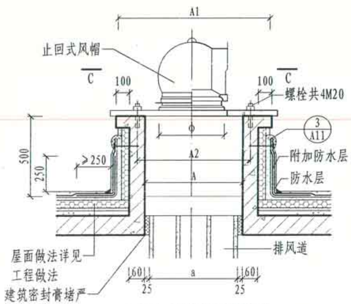
止回式风帽出屋面做法
