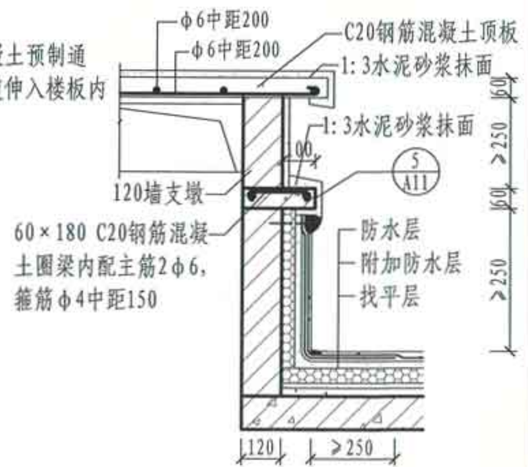
① 烟囱、通风道出屋面节点
