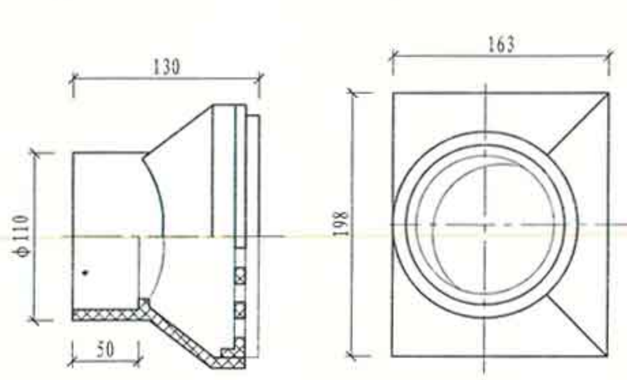
⑥ UPVC外雨水口
