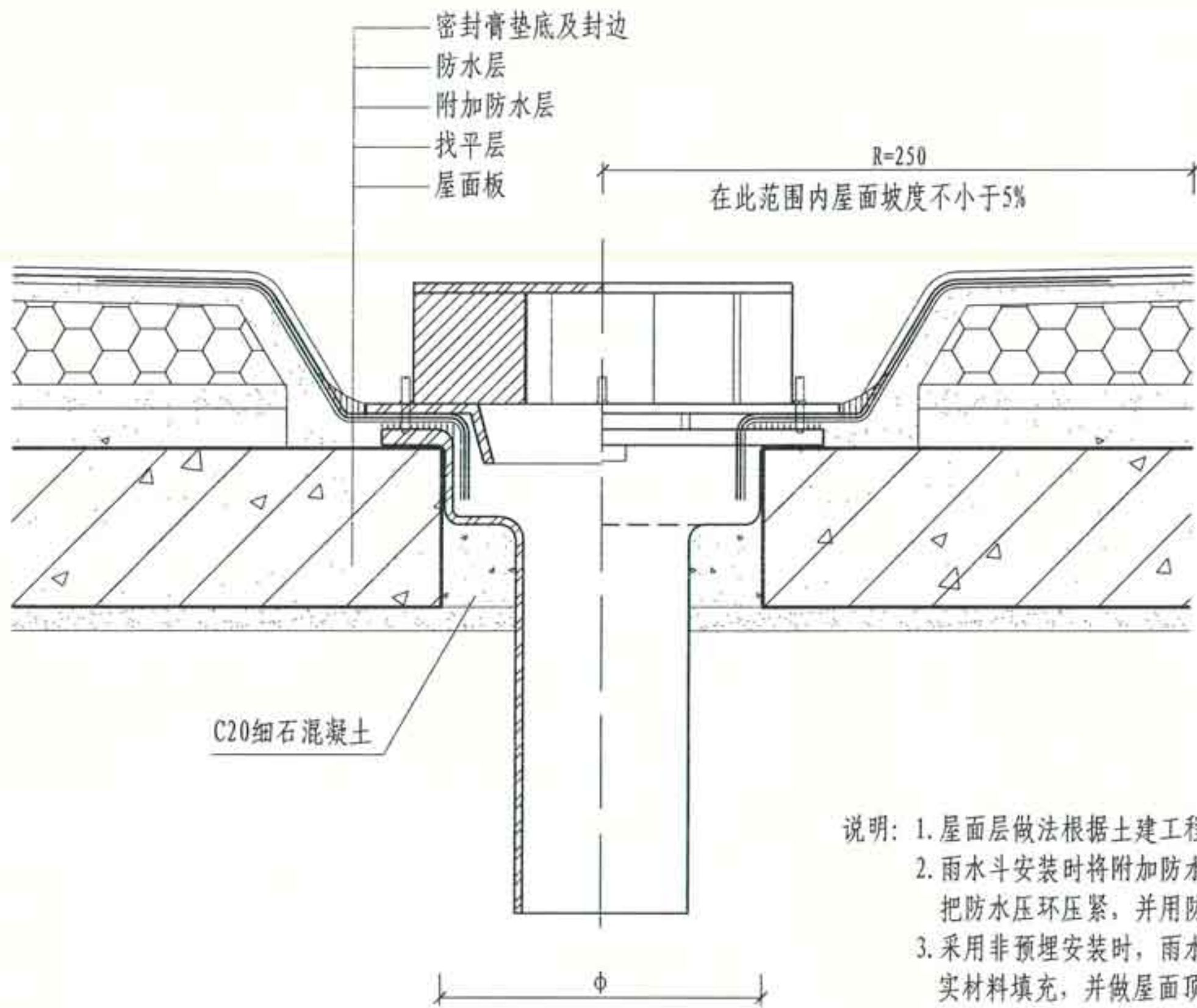
① 87改进型雨水斗安装图
