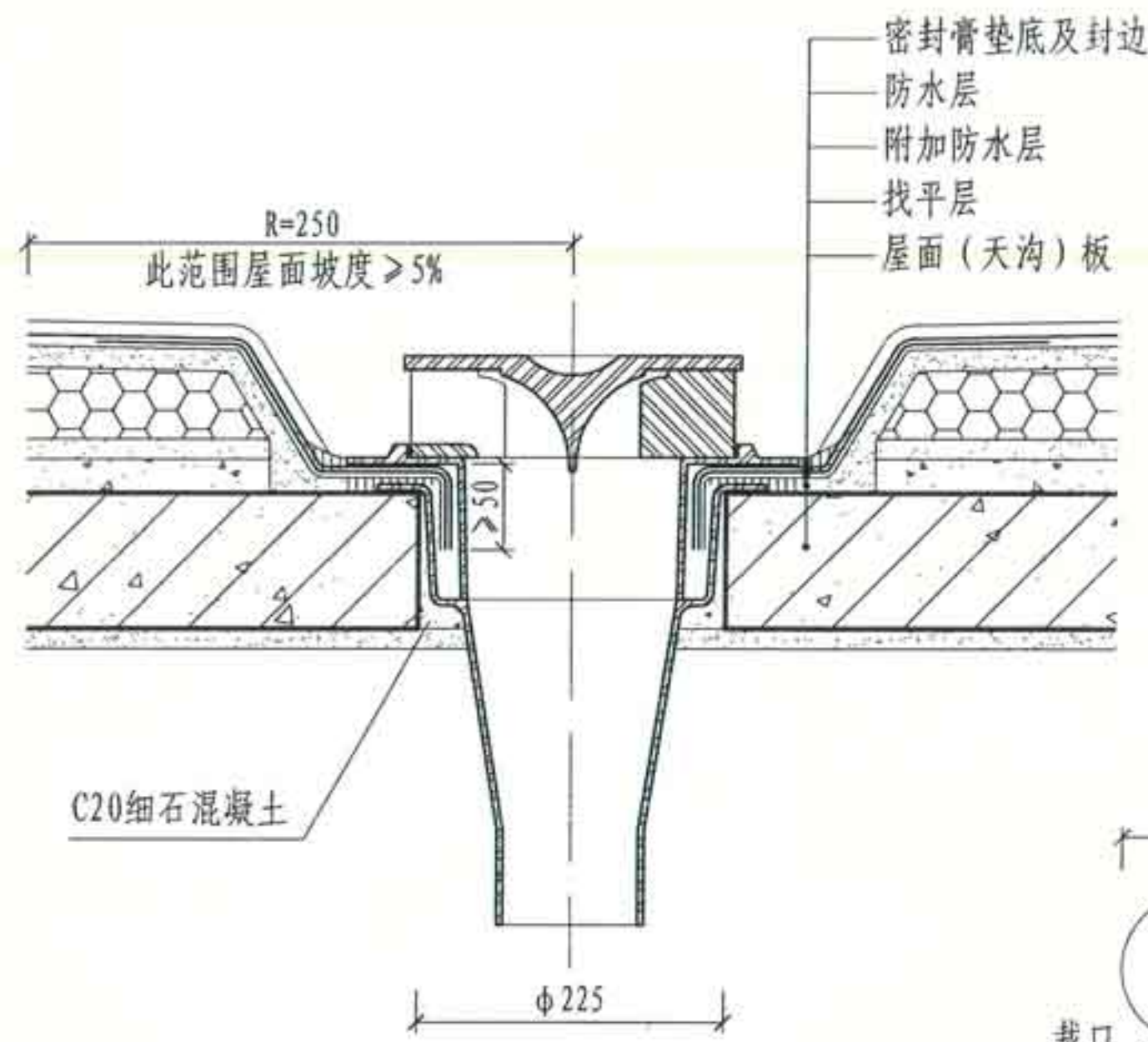
① 屋面(天沟)板上安装(一)
