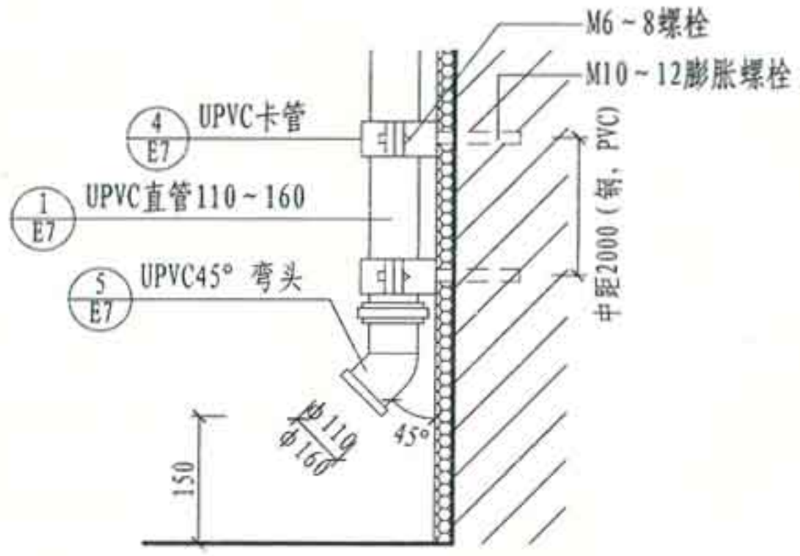
② 外排UPVC管底出水口
