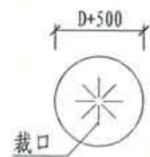
雨水口附加防水层叉面裁剪图
