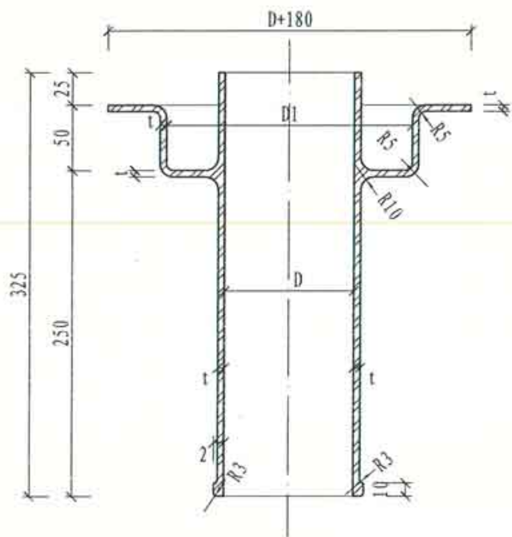
1-1剖面图
