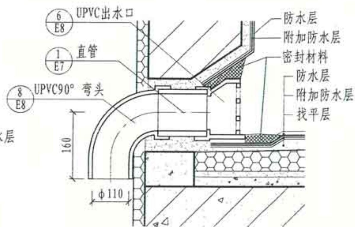
D 女儿墙UPVC雨水口
