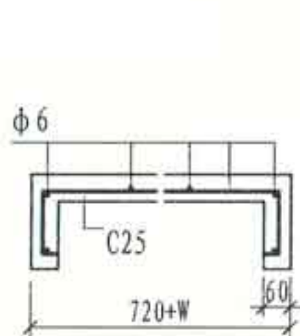
(A) 配筋图
