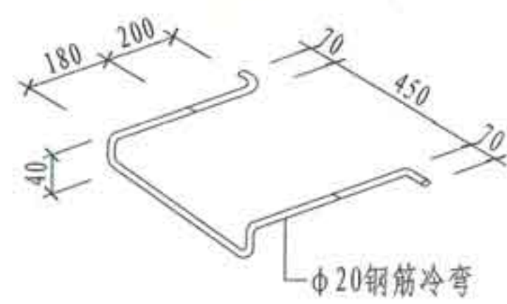
爬梯详图
