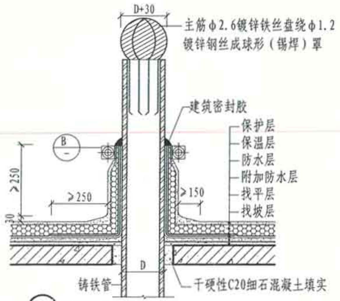
① 铸铁管出屋面
