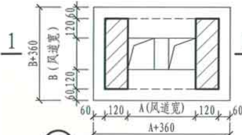
1 (双孔砌筑)
