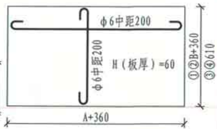
顶板构造
