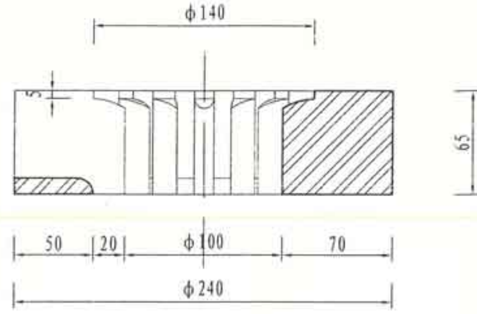
2-2剖面图
