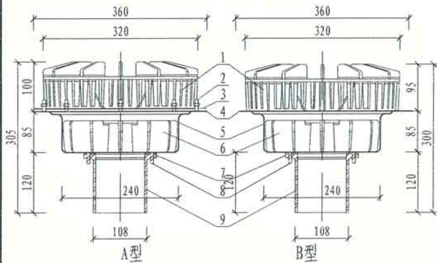
③ YG100型虹吸式雨水斗
