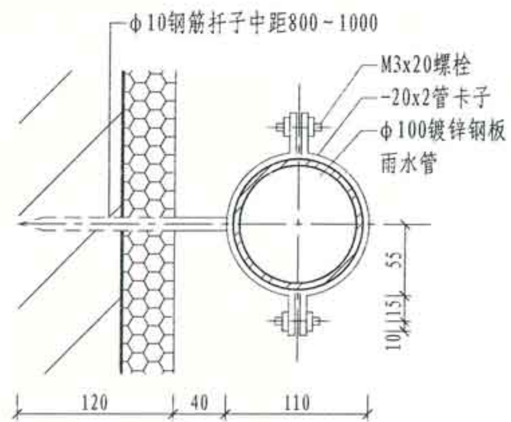
⑤ 圆雨水管及卡子
