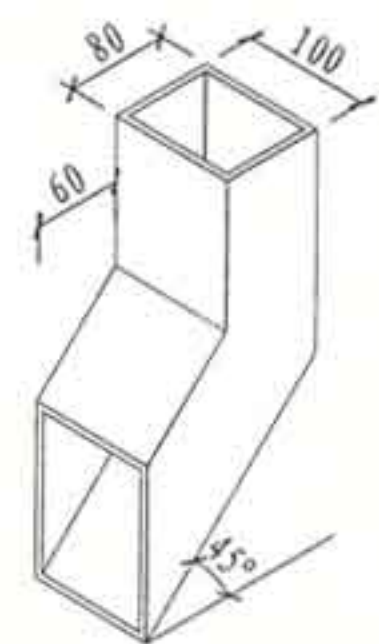
④ 外排镀锌钢板管底方(圆)出水口 注: 镀锌钢板0.6厚。
