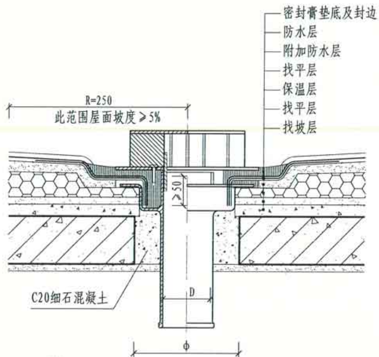
① 屋面（天沟）板上安装图
