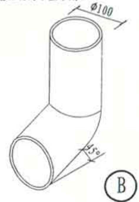
④ 外排镀锌钢板管底方(圆)出水口 注: 镀锌钢板0.6厚。
