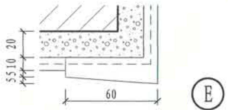
卷材、涂膜防水屋面 檐口详图
