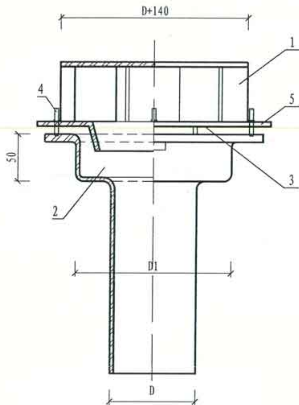
1 87改进型雨水斗装配图
