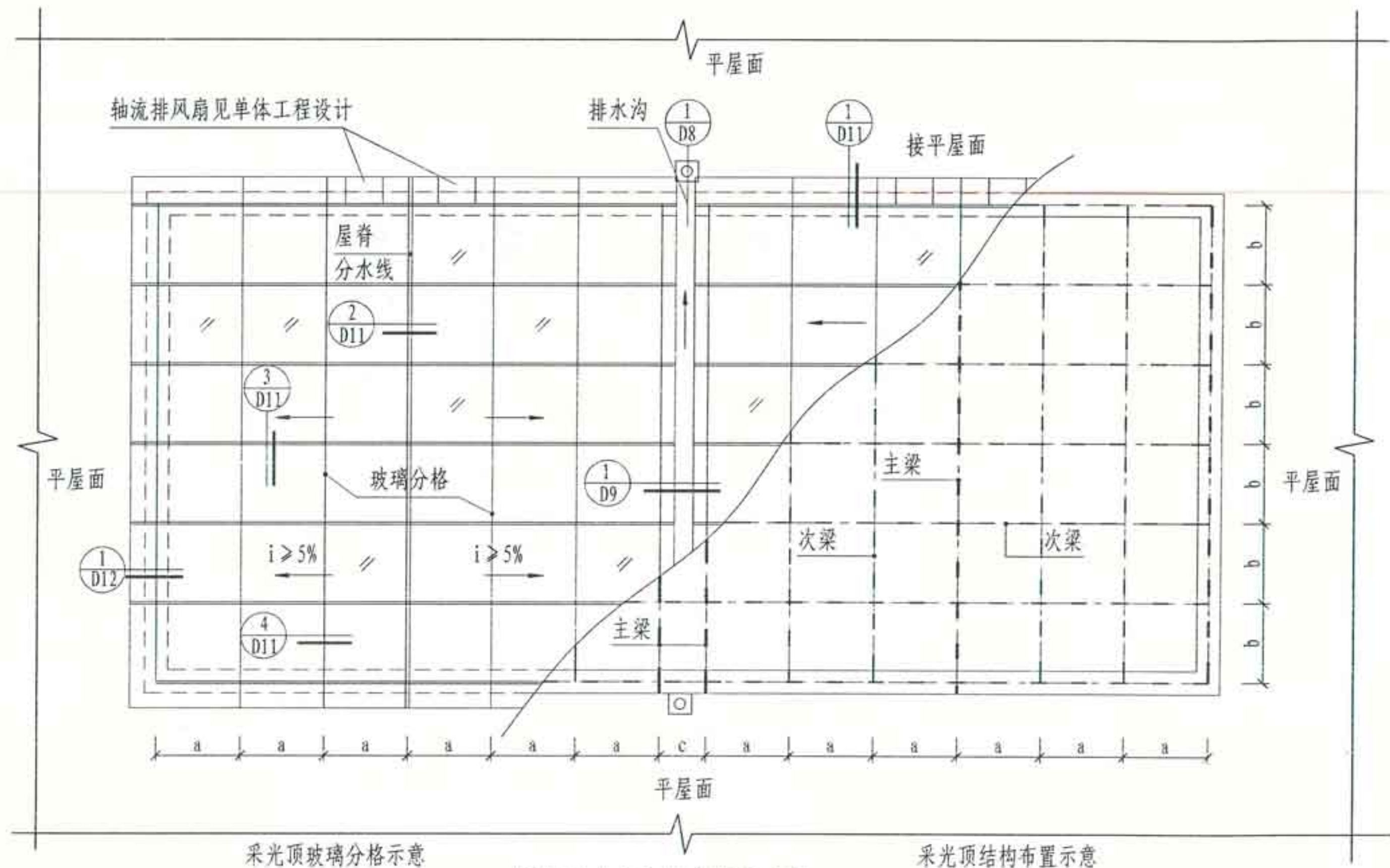
半隐框玻璃采光顶详图索引
