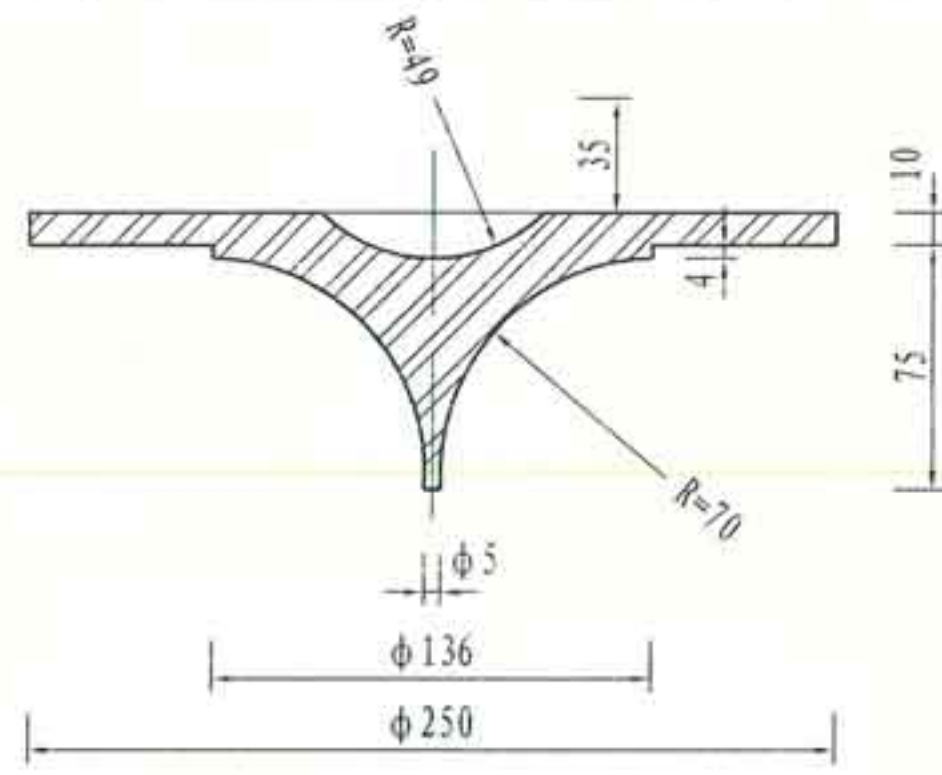
1-1剖面图
