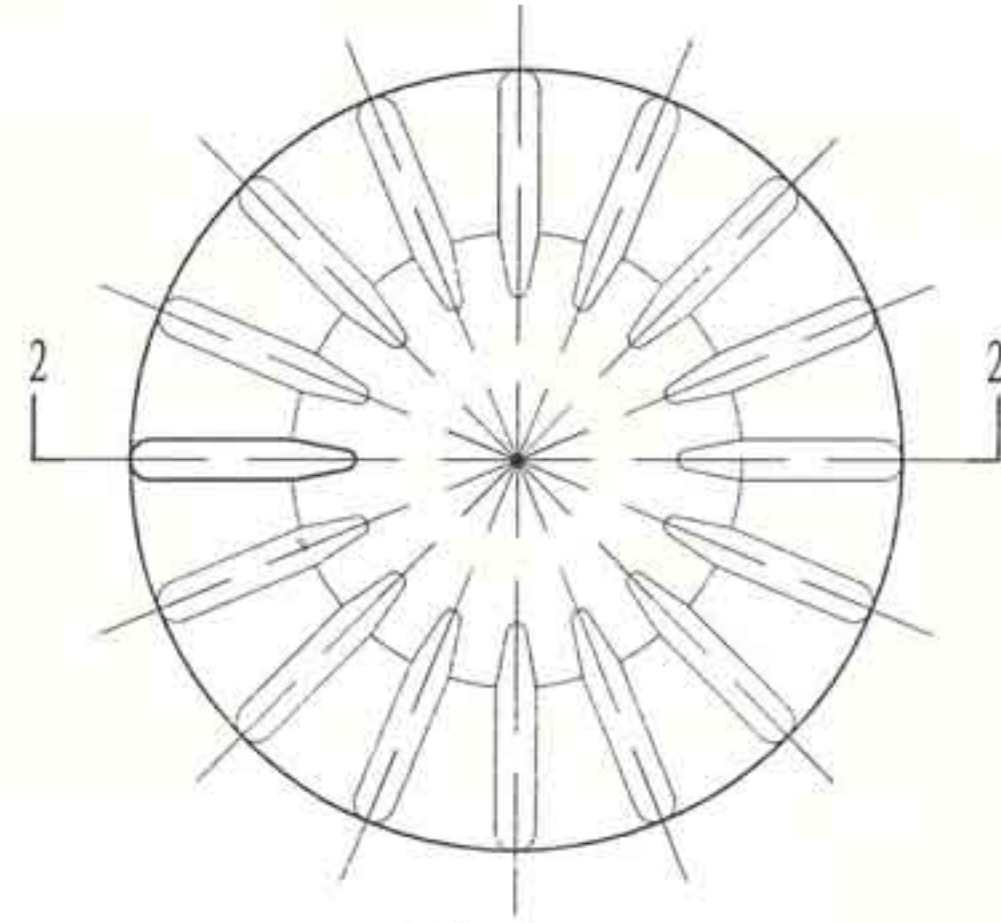
② 导流罩平面图
