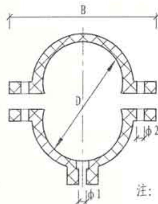
④ UPVC卡管
