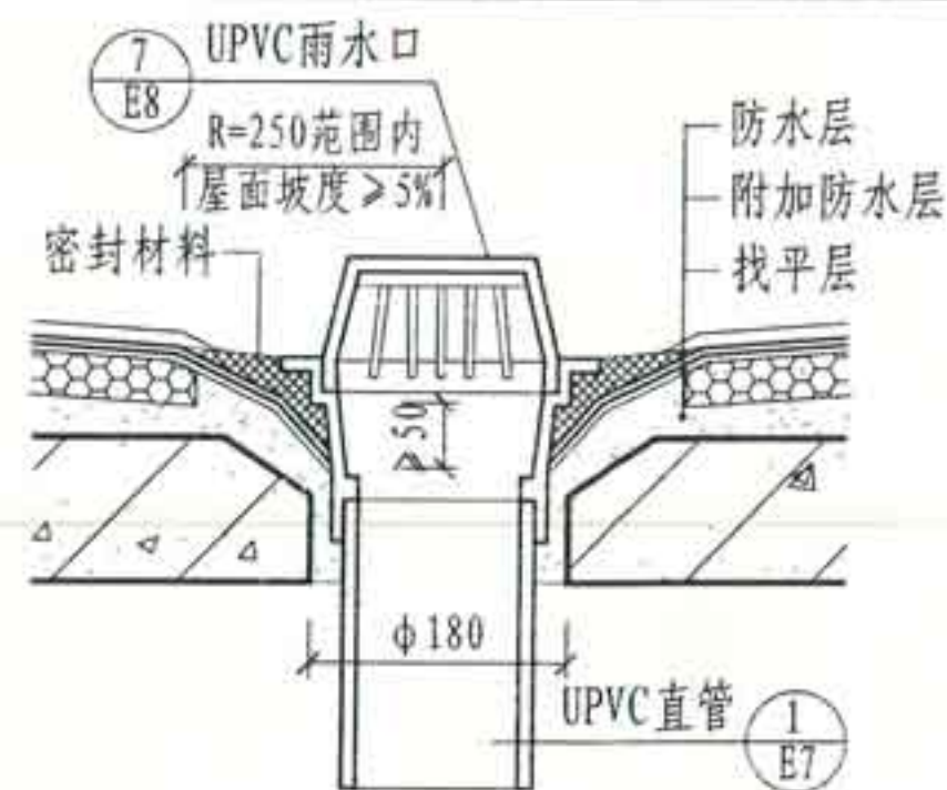
B 挑檐UPVC雨水口
