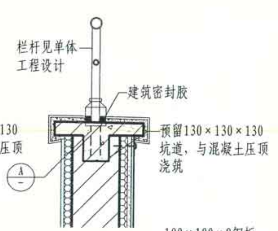
③ 栏杆
