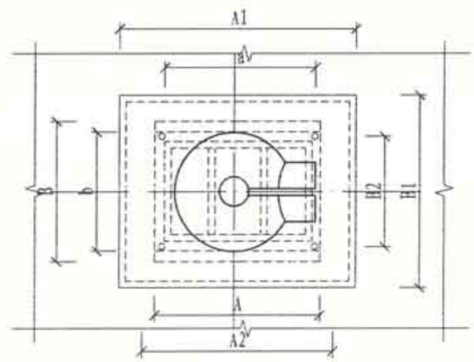
C-C止回式风帽平面图
