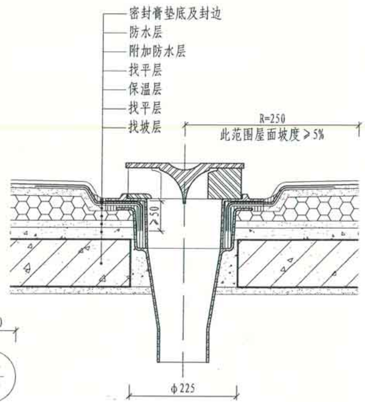
② 屋面(天沟)板上安装(二)
