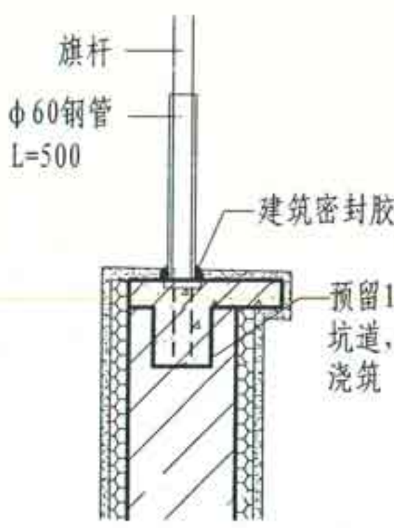
② 旗杆
