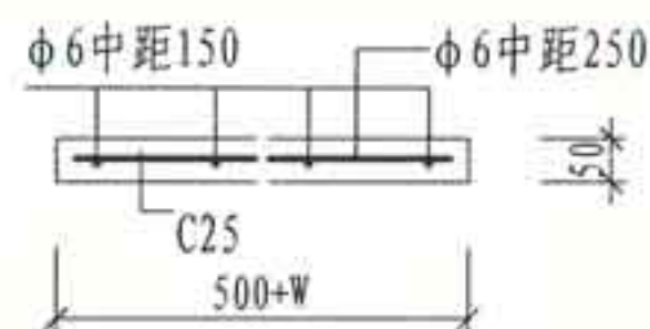
GB-1配筋图
