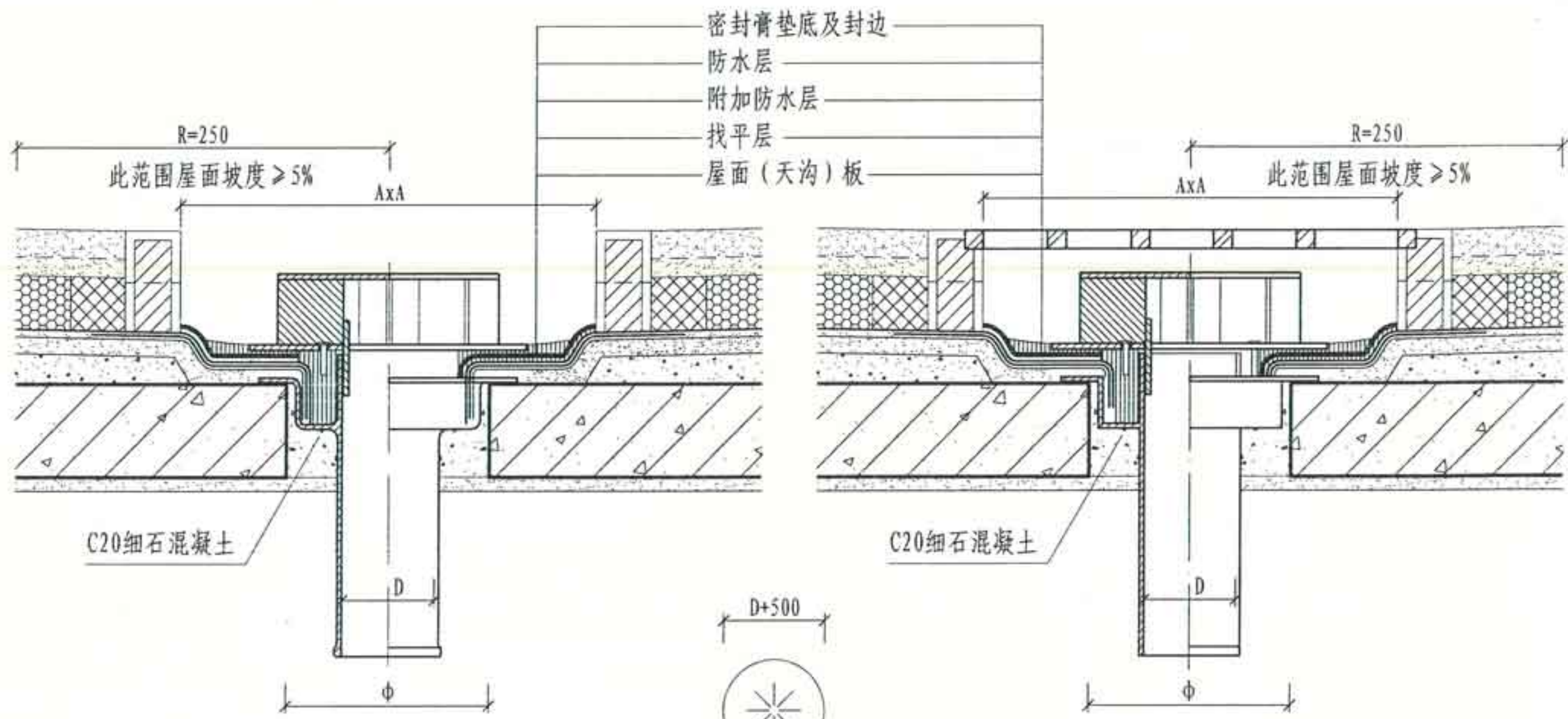
① 屋面(天沟)板上安装(I型) 用于不上人屋面
