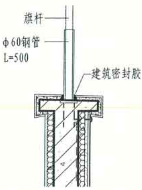
① 旗杆
