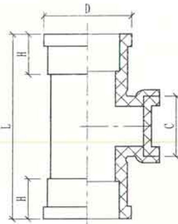
② UPVC检查口
