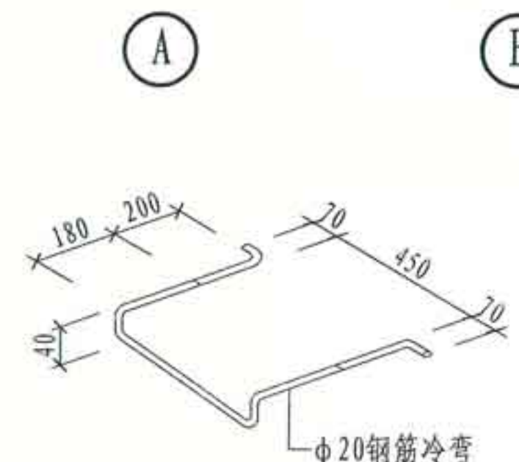
爬梯详图
