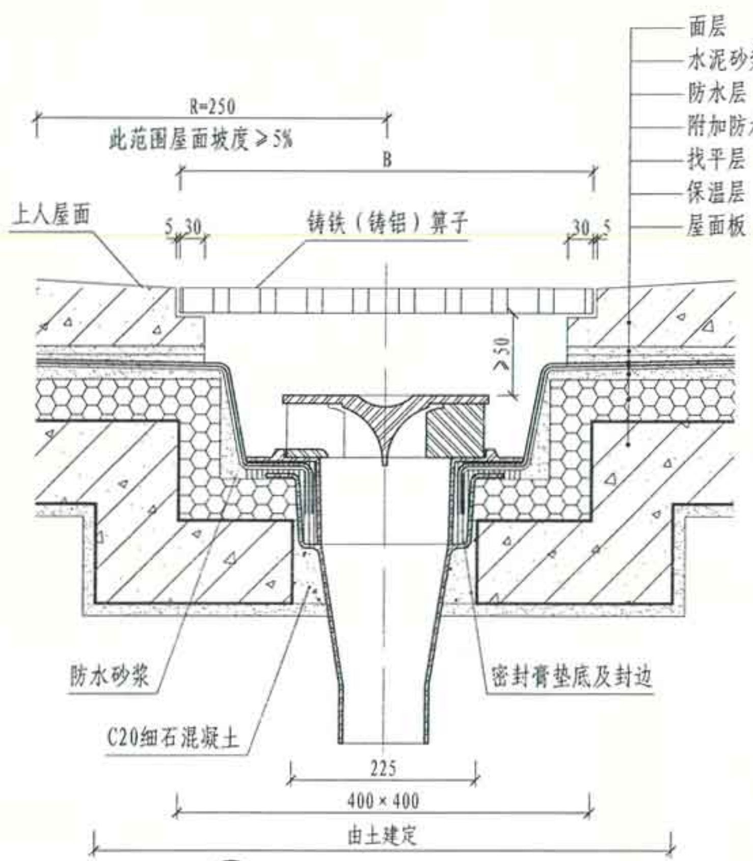
① 上人屋面雨水斗安装 (屋面板局部下凹)
