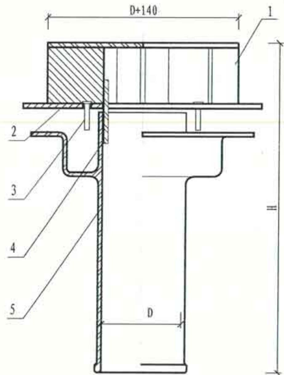
① 铸铁短管雨水斗总装配图
