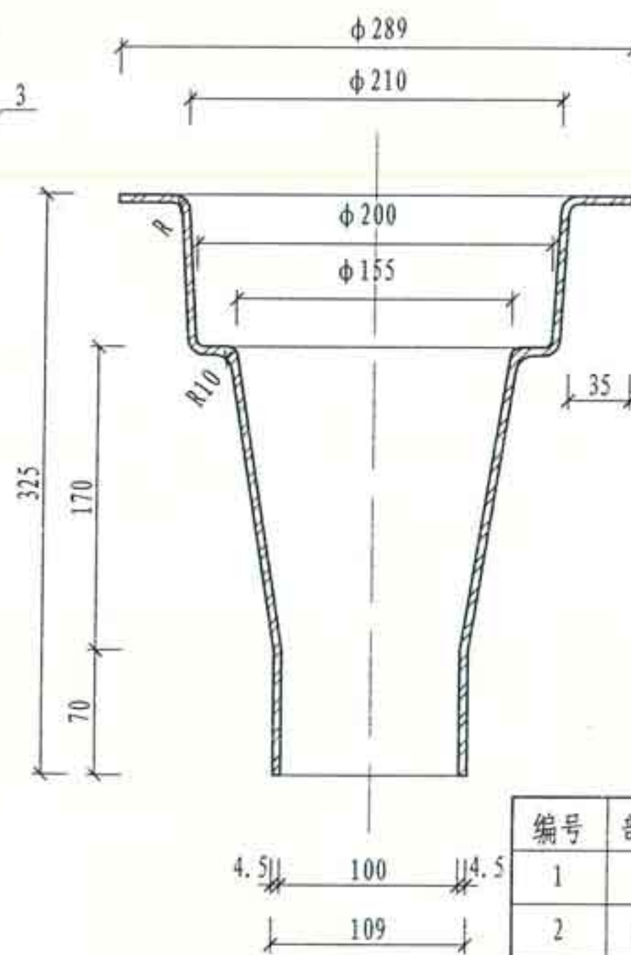
② 短管剖面图
