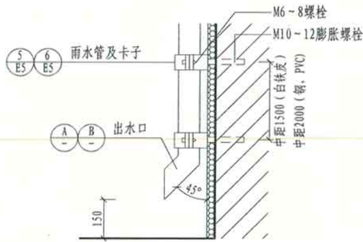
① 外排镀锌钢板管底出水口
