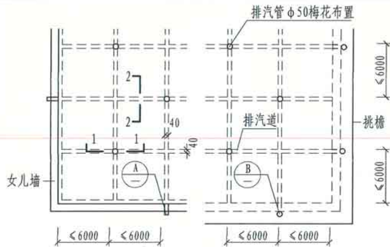
排汽道、排汽管平面布置图
