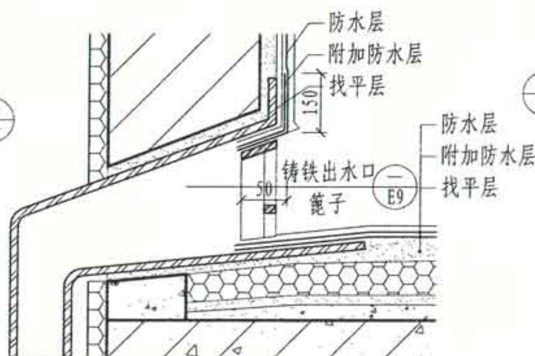
C 女儿墙铸铁雨水口
