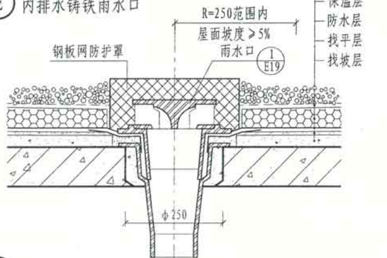
⑦ 倒置式屋面内排水雨水口
