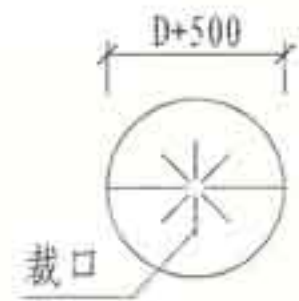
② 附加防水层叉面裁剪图
