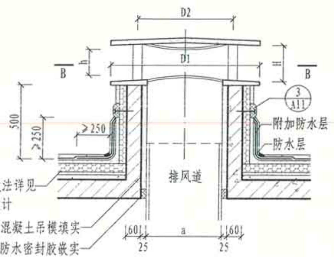
自力式风帽出屋面做法
