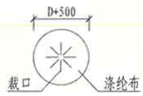
② 附加防水层叉面裁剪图
