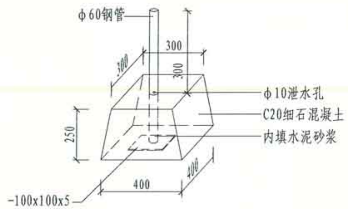
屋面旗杆座透视图
