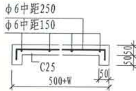
GB-1配筋图 (板长1000)
