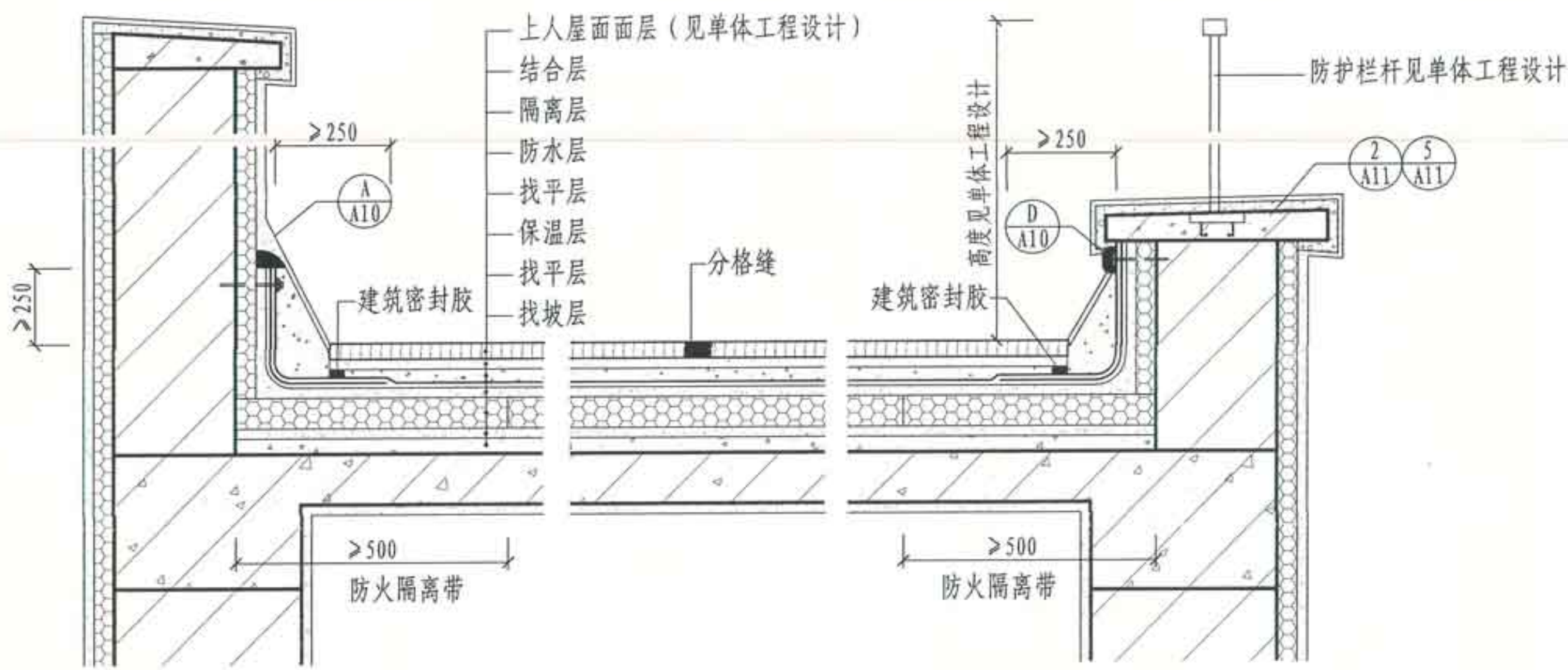
① 女儿墙处屋面泛水
