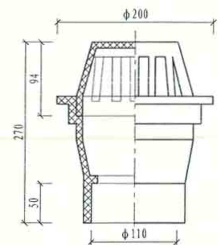
⑦ UPVC雨水口
