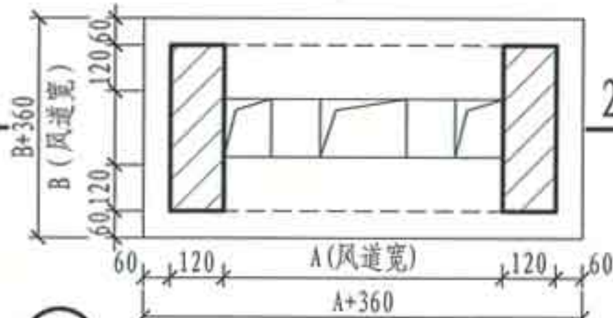
2 (三孔砌筑)
