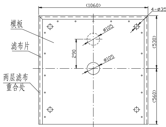
滤布片示意图 (b)
