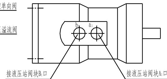
液压马达示意图
