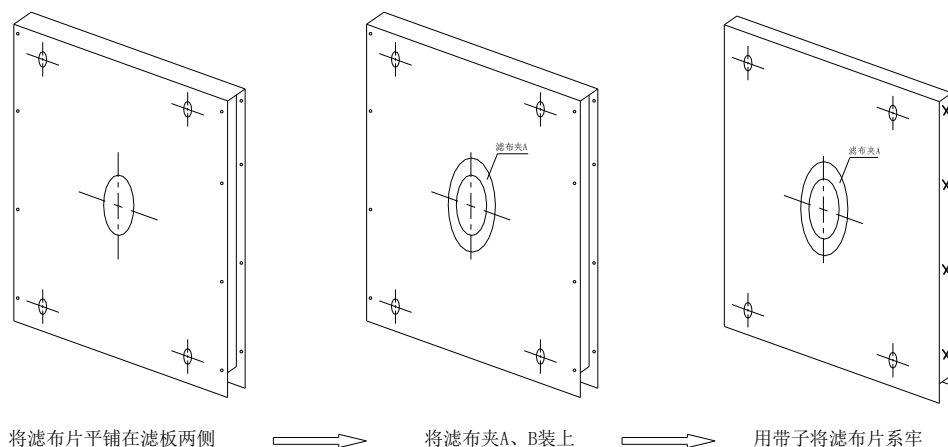
滤布片安装示意图(f)
