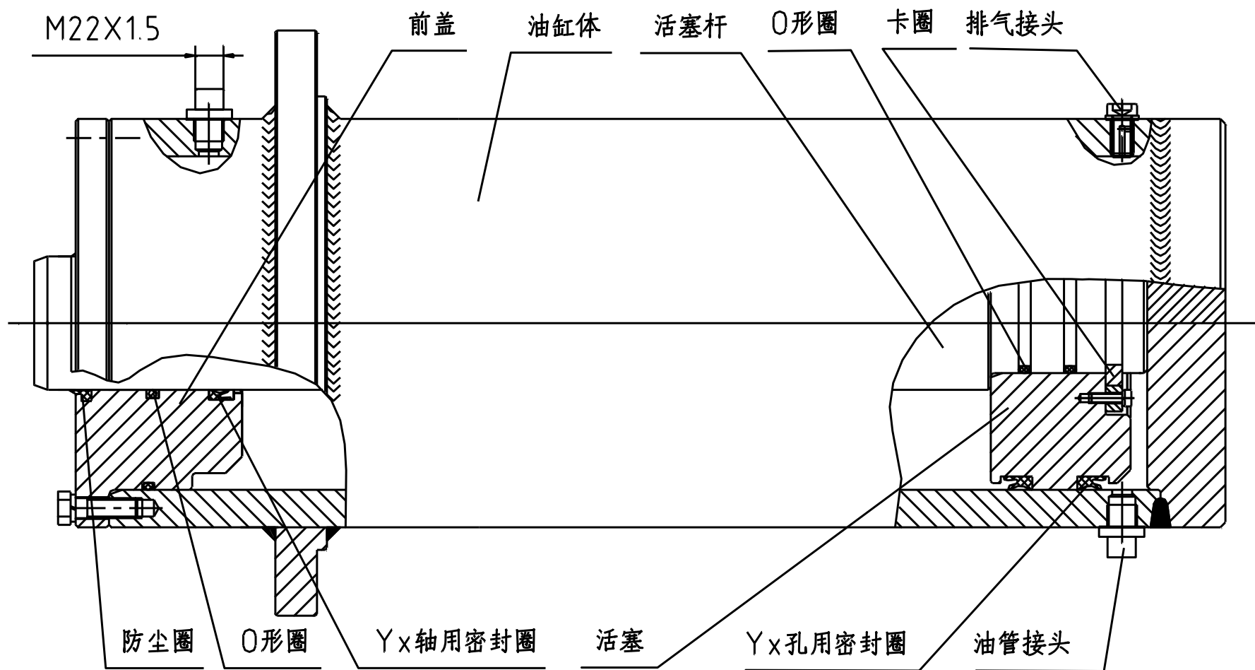
图三 油缸结构示意图(以X/1000机型油缸为例)
