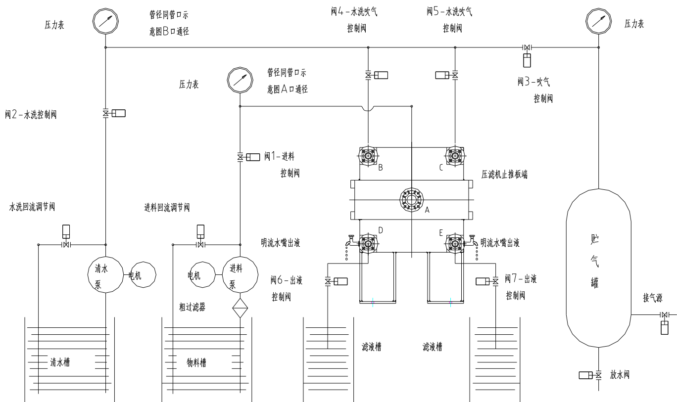
图八 管道布置图(仅供参考)
