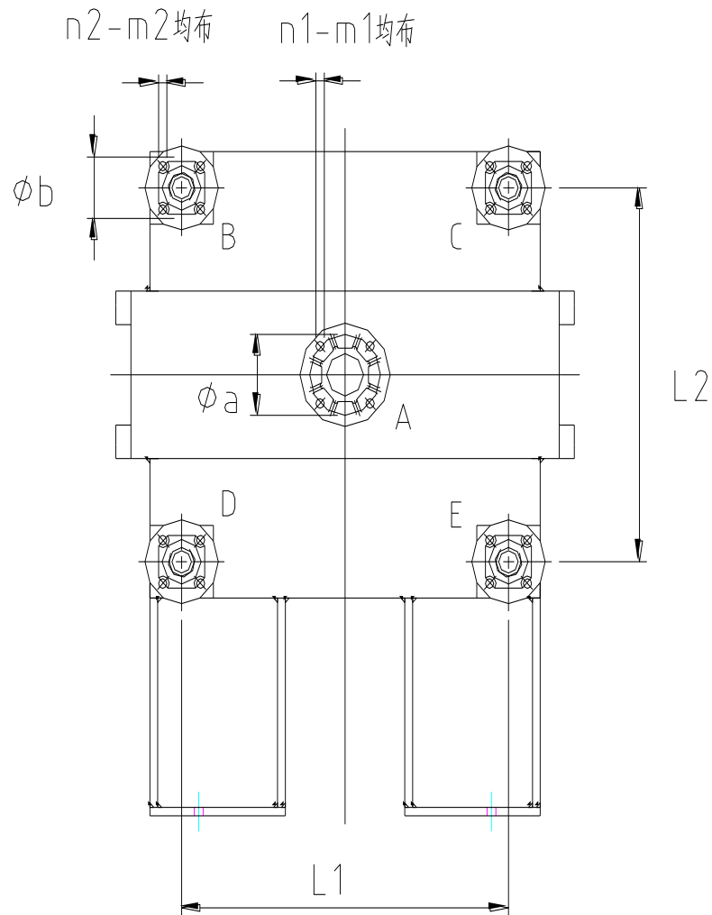
图七 管口示意图
